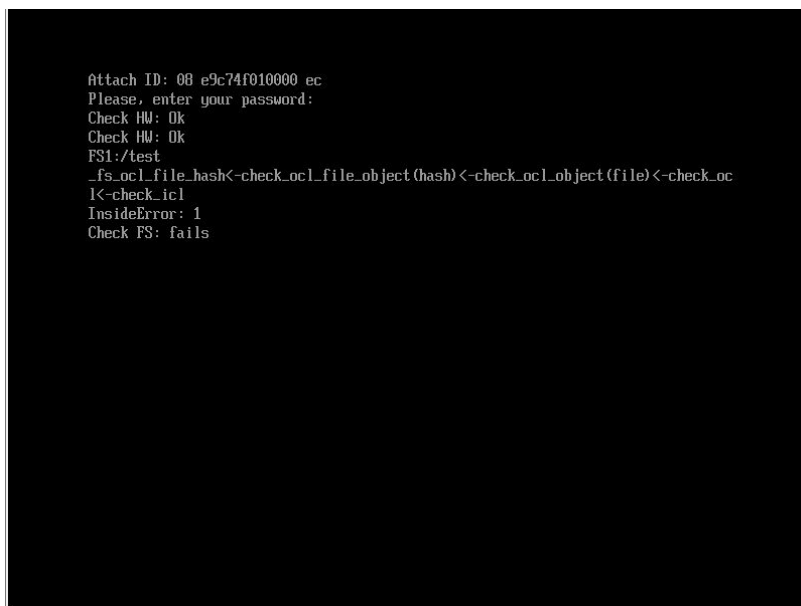
Рисунок 49 - Нарушение КЦ файлов
