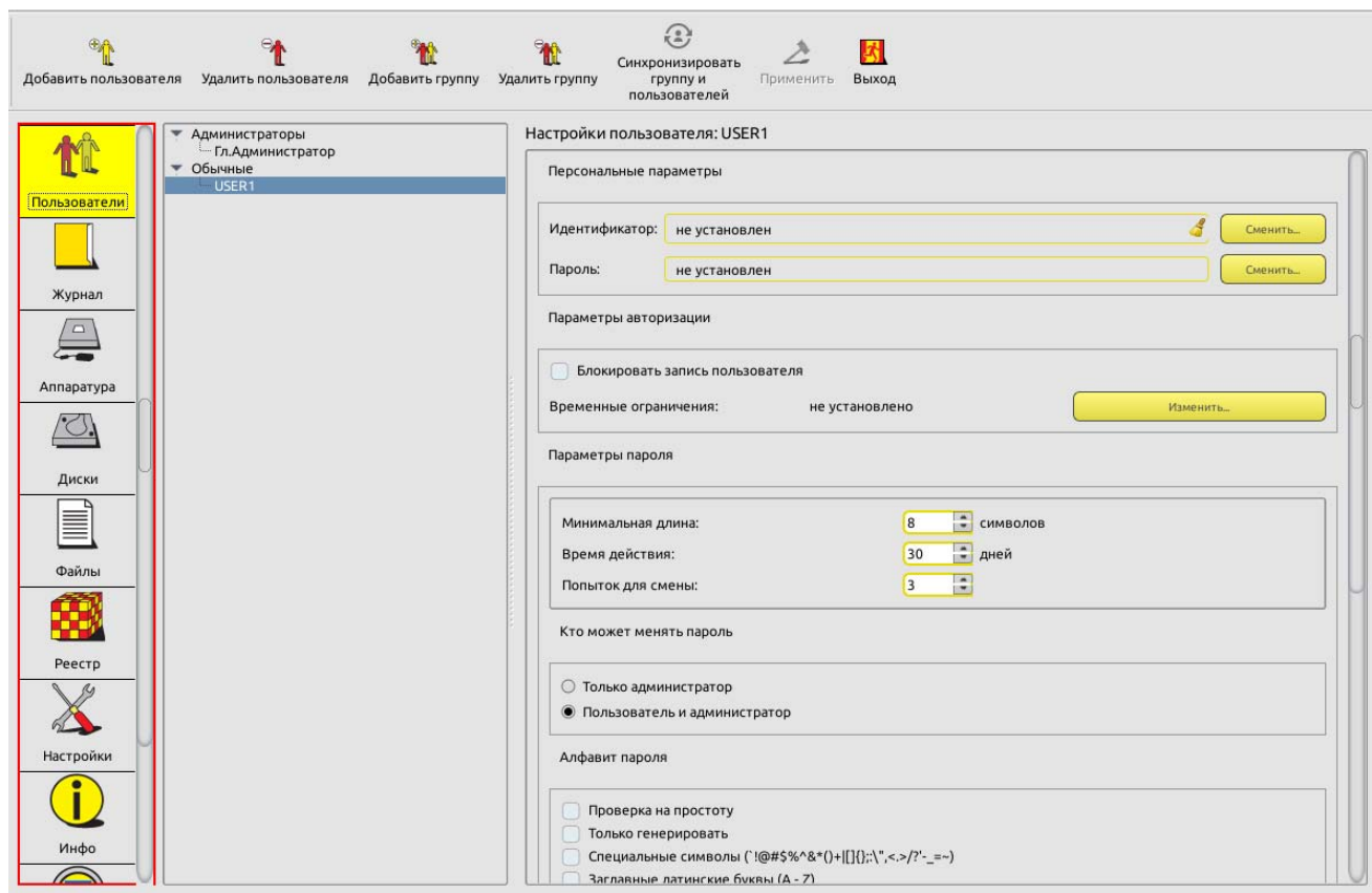
Рисунок 21 – Параметры пользователей в группе «Обычные» (для моделей Аккорд-АМДЗ» ТУ 4012-038-11443195-2011, ТУ 26.20.40.140-079-37222406-2019 и ТУ 26.20.40.140-113-РДСУ-2023)
