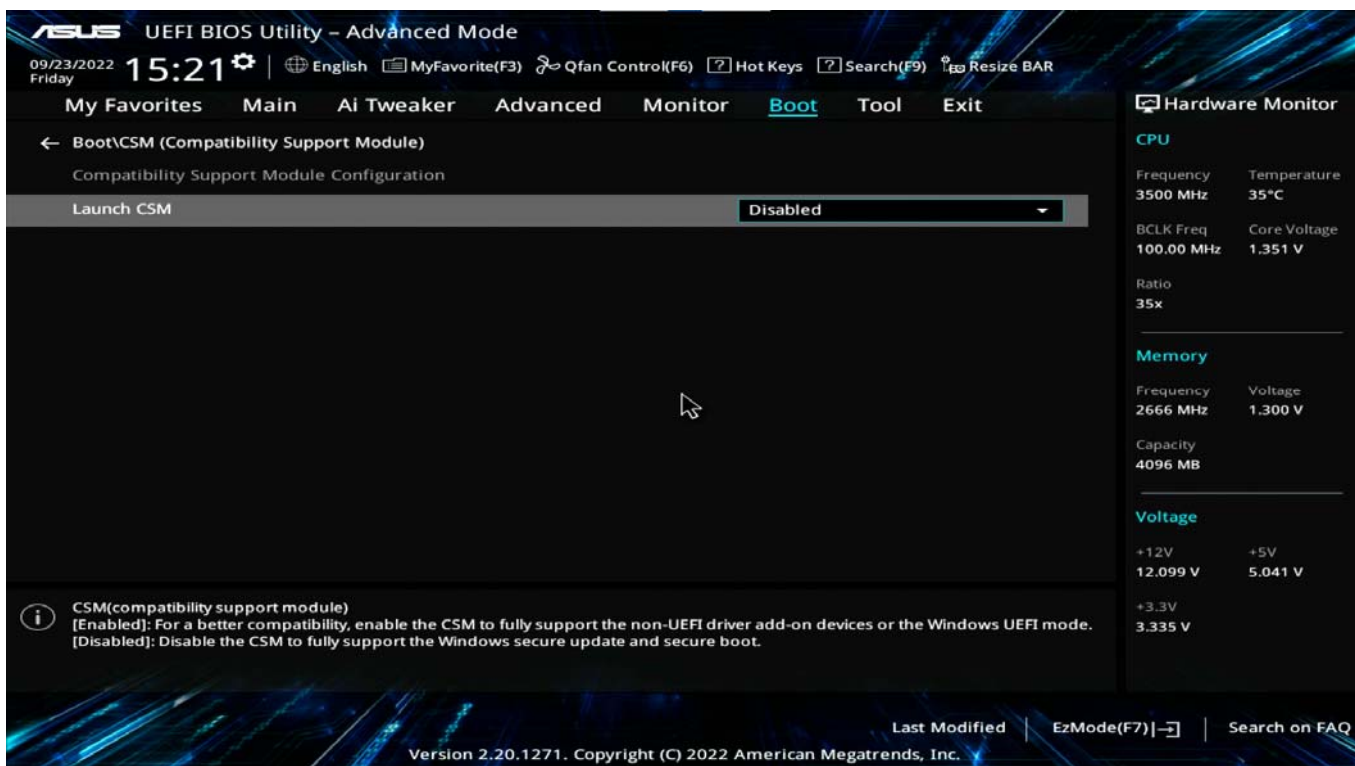
Рисунок 51 - Отключение модуля CSM
