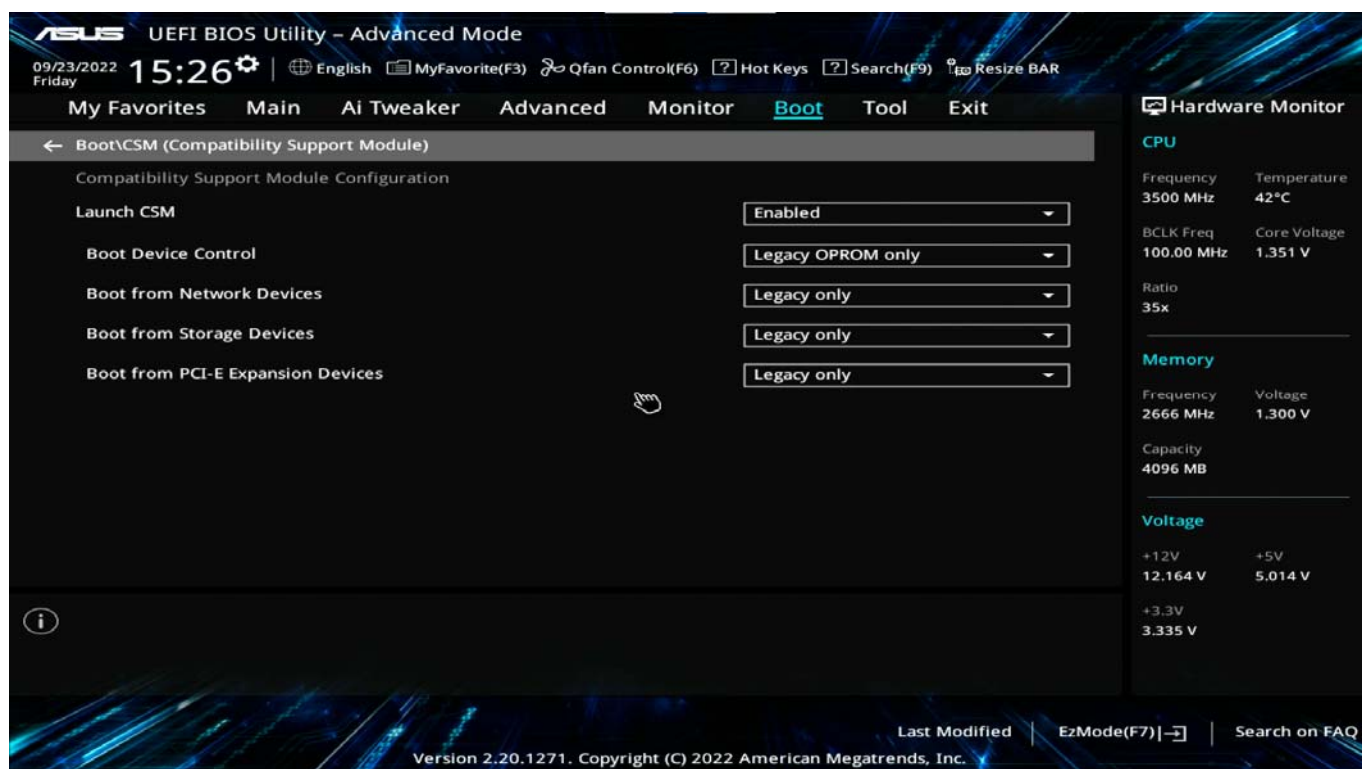
Рисунок 55 - Проверка значения модуля CSM
