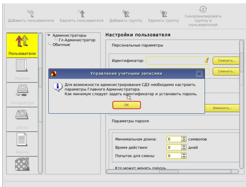
Рисунок 44 - Старт среды администрирования
