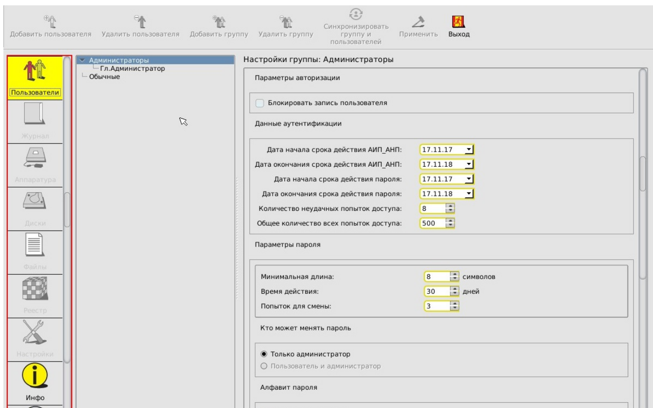
Рисунок 2 - Главное окно среды администрирования (для моделей Аккорд-АМДЗ» ТУ 4012-054-11443195-2013, ТУ 26.20.40.140-097-37222406-2021, ТУ 26.20.40.140-108-37222406-2022 и ТУ 26.20.40.140-115-37222406-2023)
