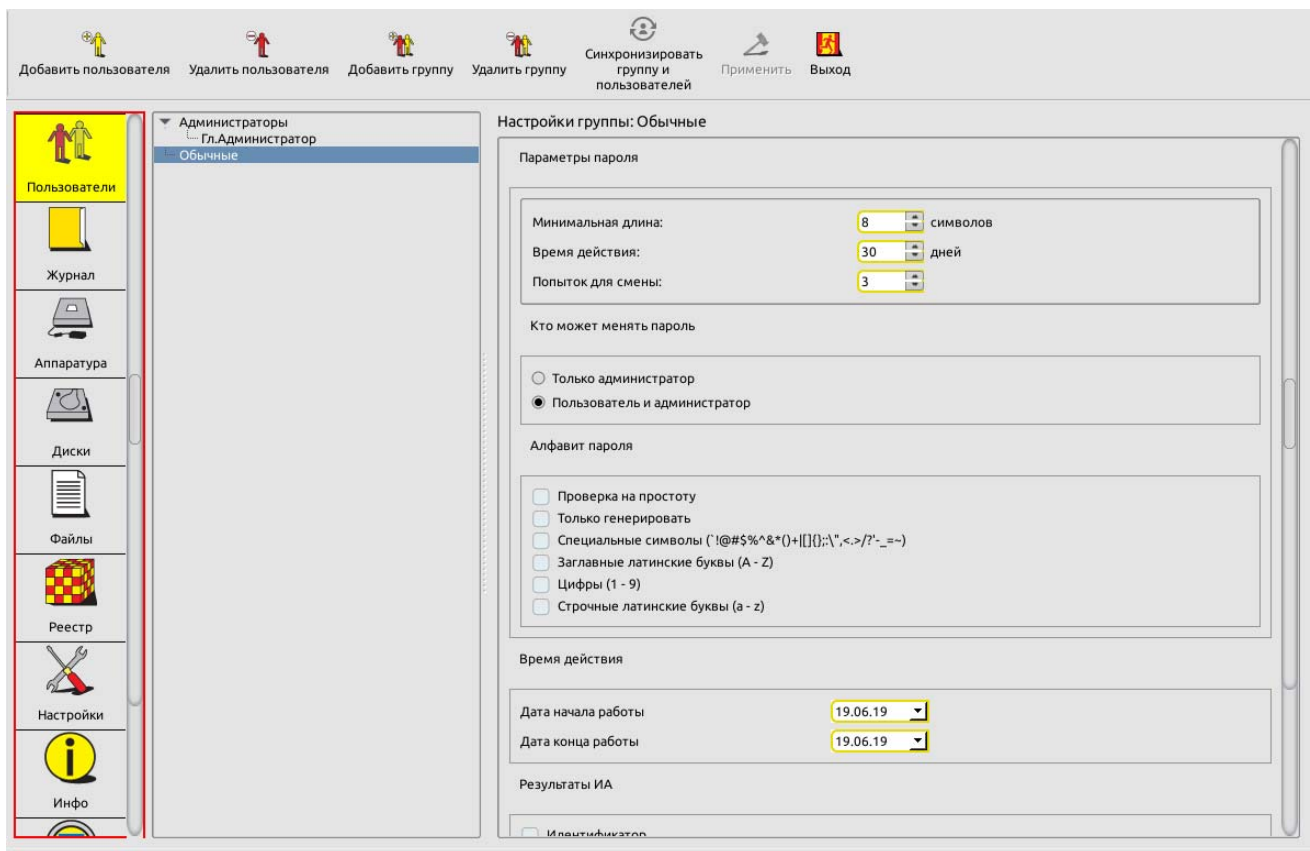
Рисунок 16 – Общие параметры группы «Обычные» (для моделей Аккорд-АМДЗ» ТУ 4012-038-11443195-2011, ТУ 26.20.40.140-079-37222406-2019 и ТУ 26.20.40.140- 113-РДСУ-2023)
