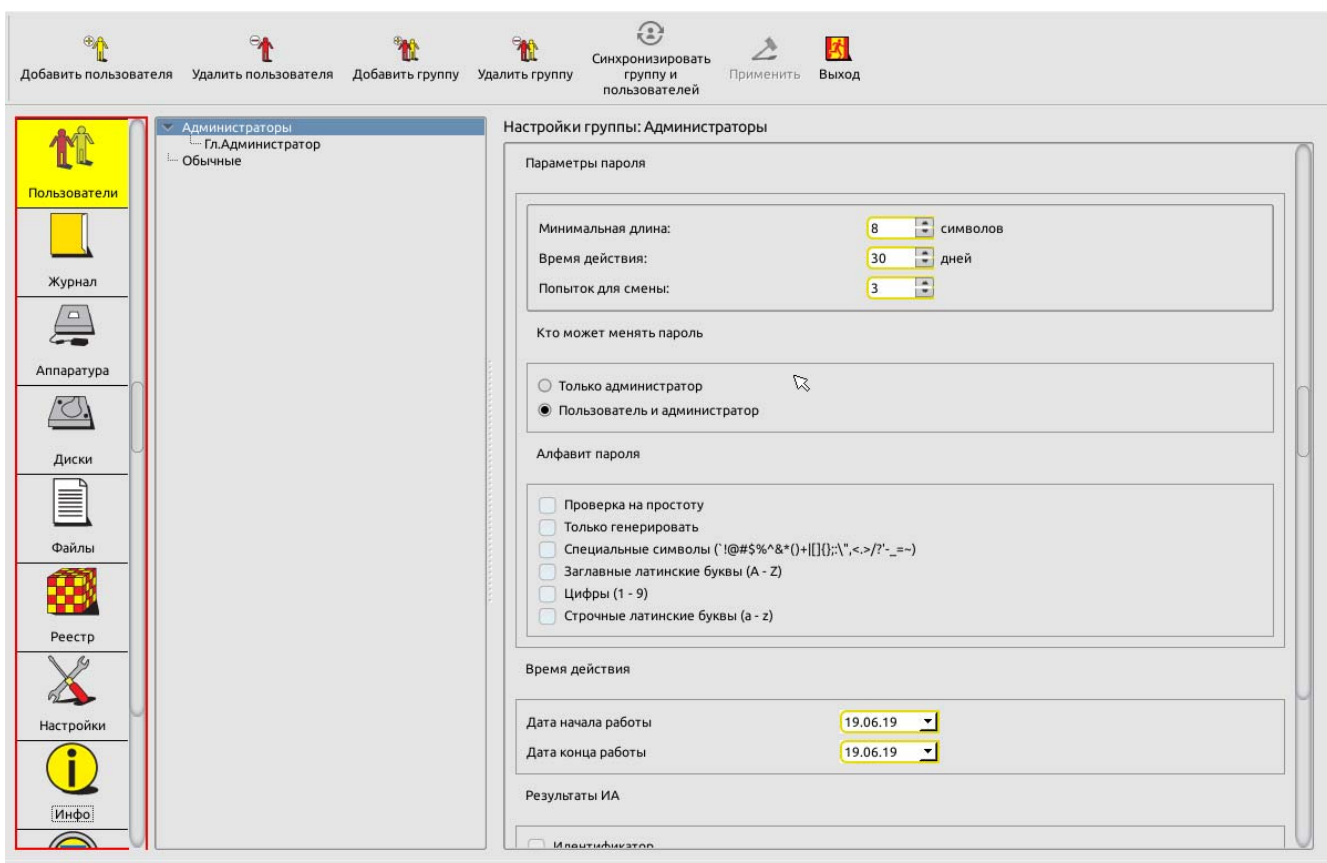
Рисунок 14 - Общие параметры группы «Администраторы» (для моделей Аккорд-АМДЗ» ТУ 4012-038-11443195-2011, ТУ 26.20.40.140-079-37222406-2019 и ТУ 26.20.40.140-113-РДСУ-2023)
