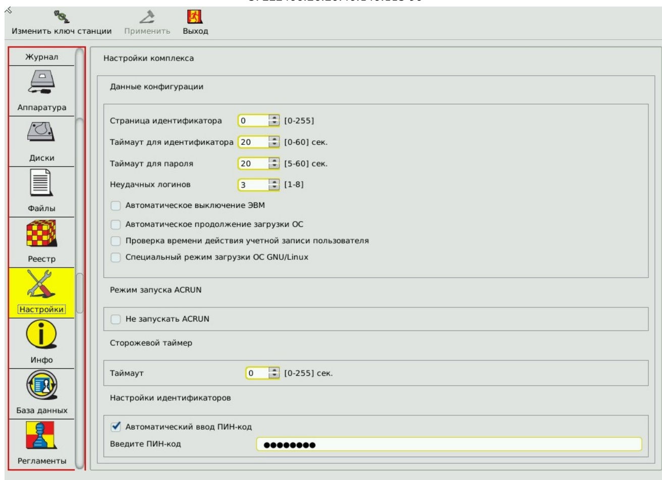
Рисунок 36 - Общие настройки комплекса (для моделей Аккорд-АМДЗ» ТУ 4012-054-11443195-2013, ТУ 26.20.40.140-097-37222406-2021, ТУ 26.20.40.140-108-37222406-2022 и ТУ 26.20.40.140-115-37222406-2023)
