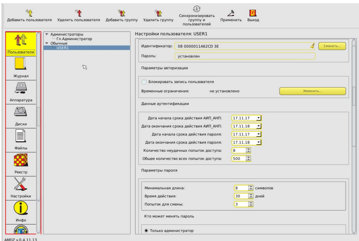
Рисунок 22 - Параметры пользователей в группе «Обычные» (для моделей Аккорд-АМДЗ» ТУ 4012-054-11443195-2013, ТУ 26.20.40.140-097-37222406-2021, ТУ 26.20.40.140-108-37222406-2022 и ТУ 26.20.40.140-115-37222406-2023)
