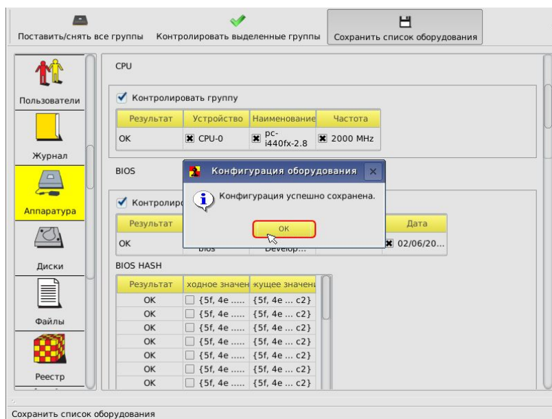
Рисунок 47 - Установка на контроль аппаратуры и сохранение конфигурации
