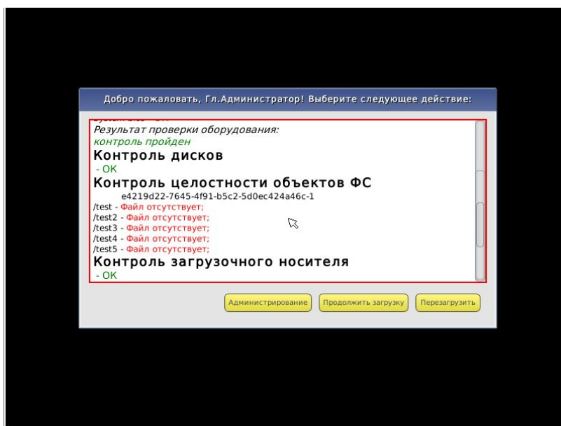
Рисунок 50 - Полный список файлов, не прошедших КЦ
