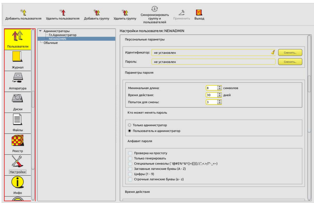
Рисунок 18 – Параметры пользователей в группе «Администраторы» (для моделей Аккорд-АМДЗ» ТУ 4012-038-11443195-2011, ТУ 26.20.40.140-079-37222406-2019 и ТУ 26.20.40.140-113-РДСУ-2023)
