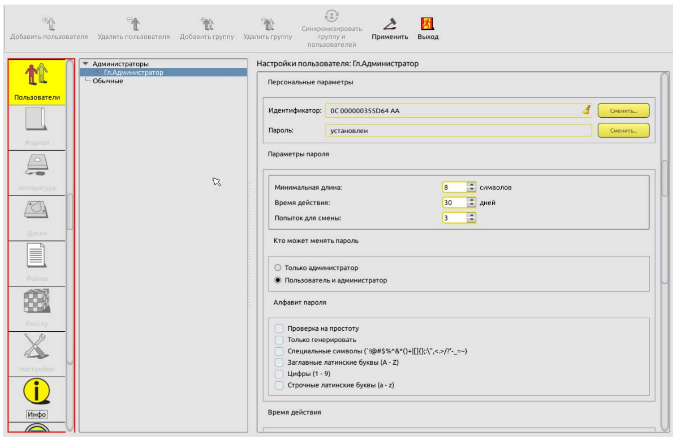
Рисунок 12 - Пароль учетной записи «Гл. Администратор» установлен (для моделей Аккорд-АМДЗ» ТУ 4012-038-11443195-2011, ТУ 26.20.40.140-079-37222406-2019 и ТУ 26.20.40.140-113-РДСУ-2023)
