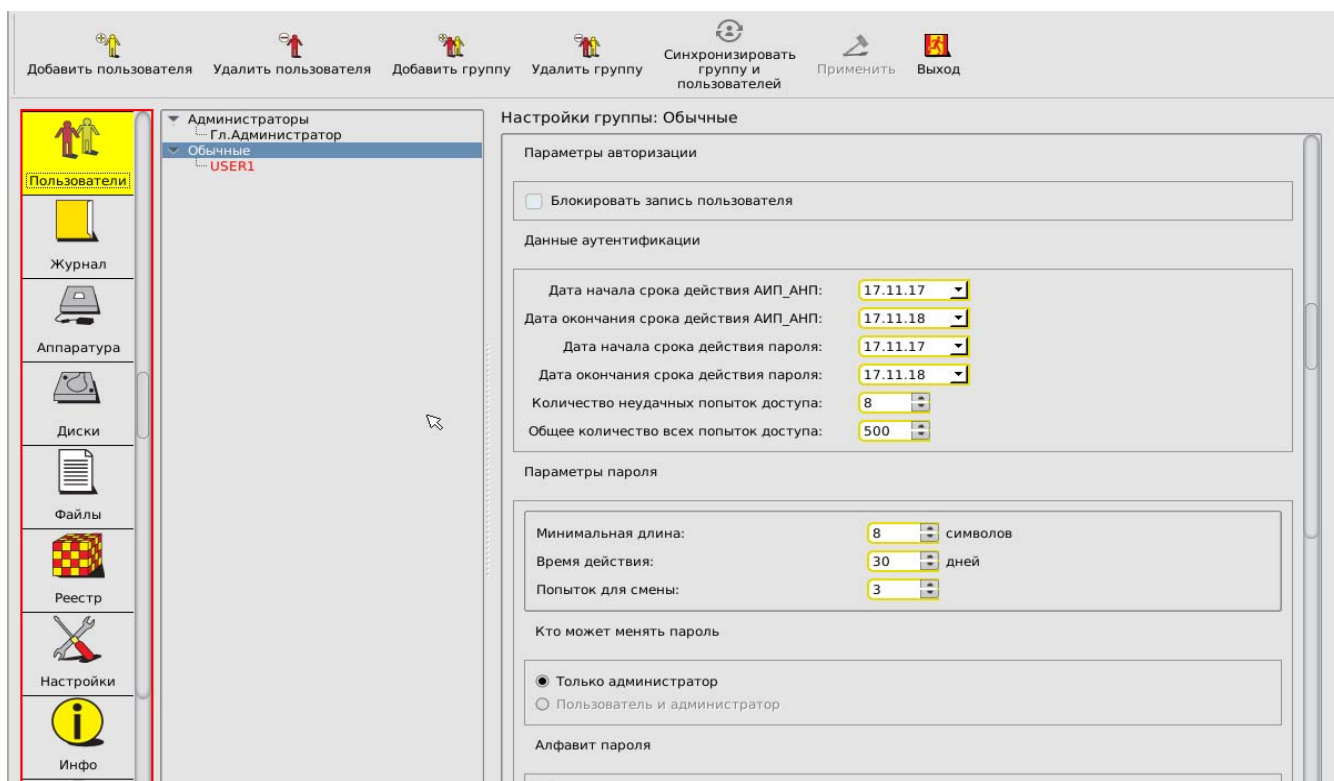
Рисунок 17 - Общие параметры группы «Обычные» (для моделей Аккорд-АМДЗ» ТУ 4012-054-11443195-2013, ТУ 26.20.40.140-097-37222406-2021, ТУ 26.20.40.140-108-37222406-2022 и ТУ 26.20.40.140-115-37222406-2023)
