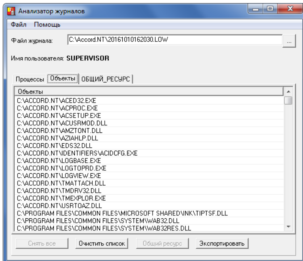
Рисунок 92 – Главное окно программы AcProc.exe. Вкладка «Объекты»
