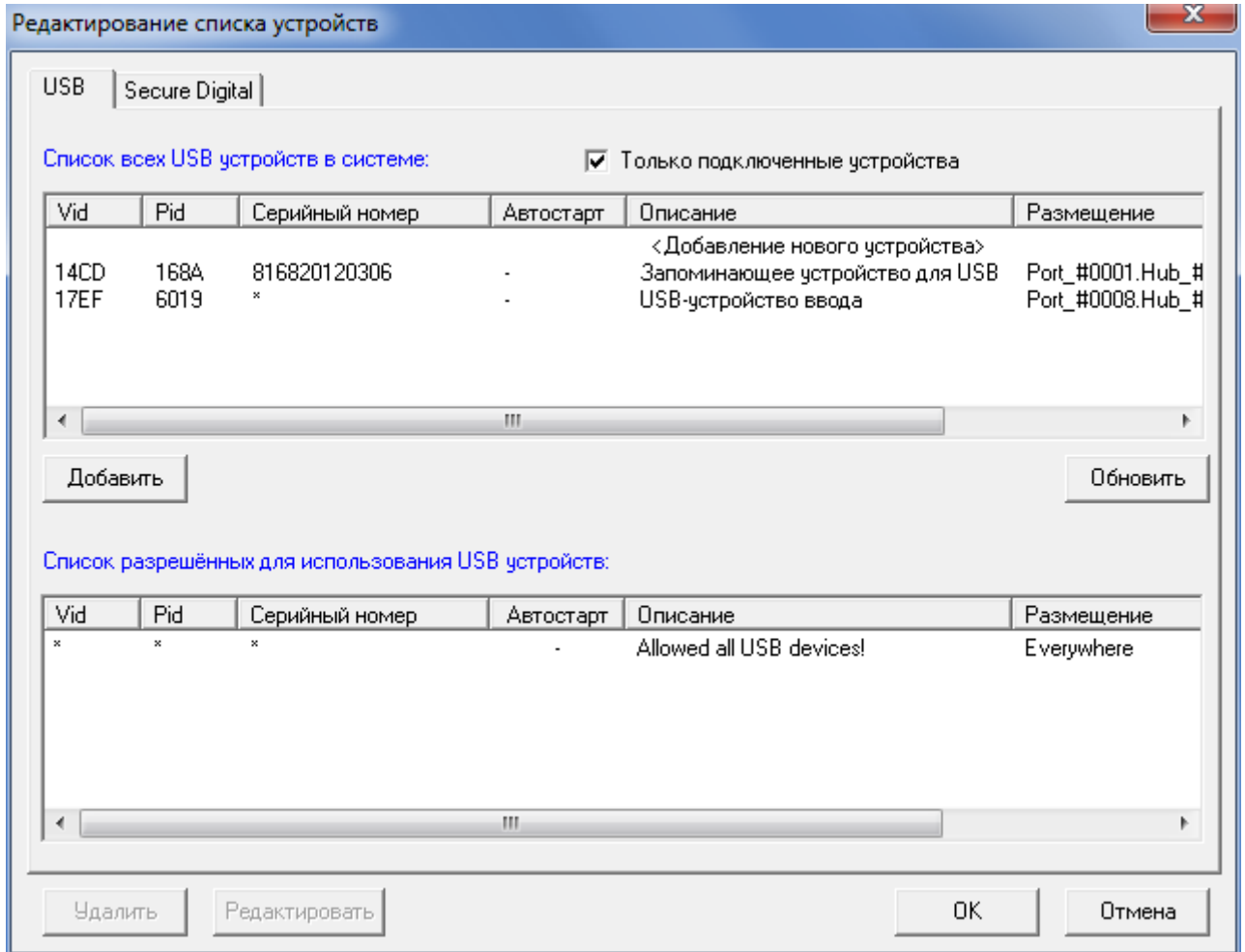
Рисунок 114 - Окно редактирования списка разрешенных USB устройств
