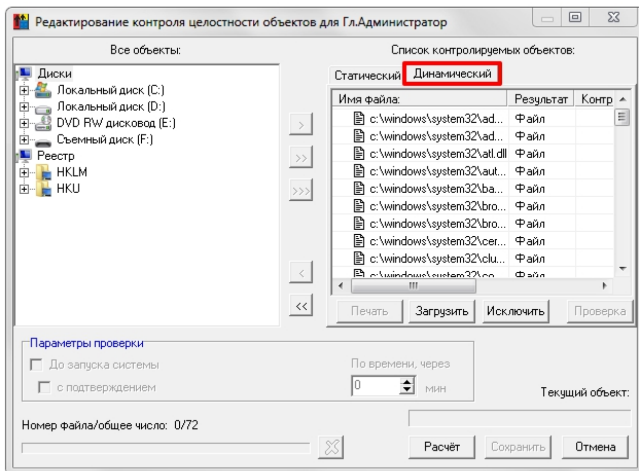
Рисунок 102 - Редактирование списков для контроля целостности. Импорт списка контролируемых объектов
