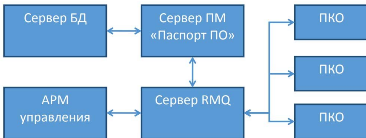
Рисунок 1 - Основные элементы ПМ «Паспорт ПО» и их взаимодействие
