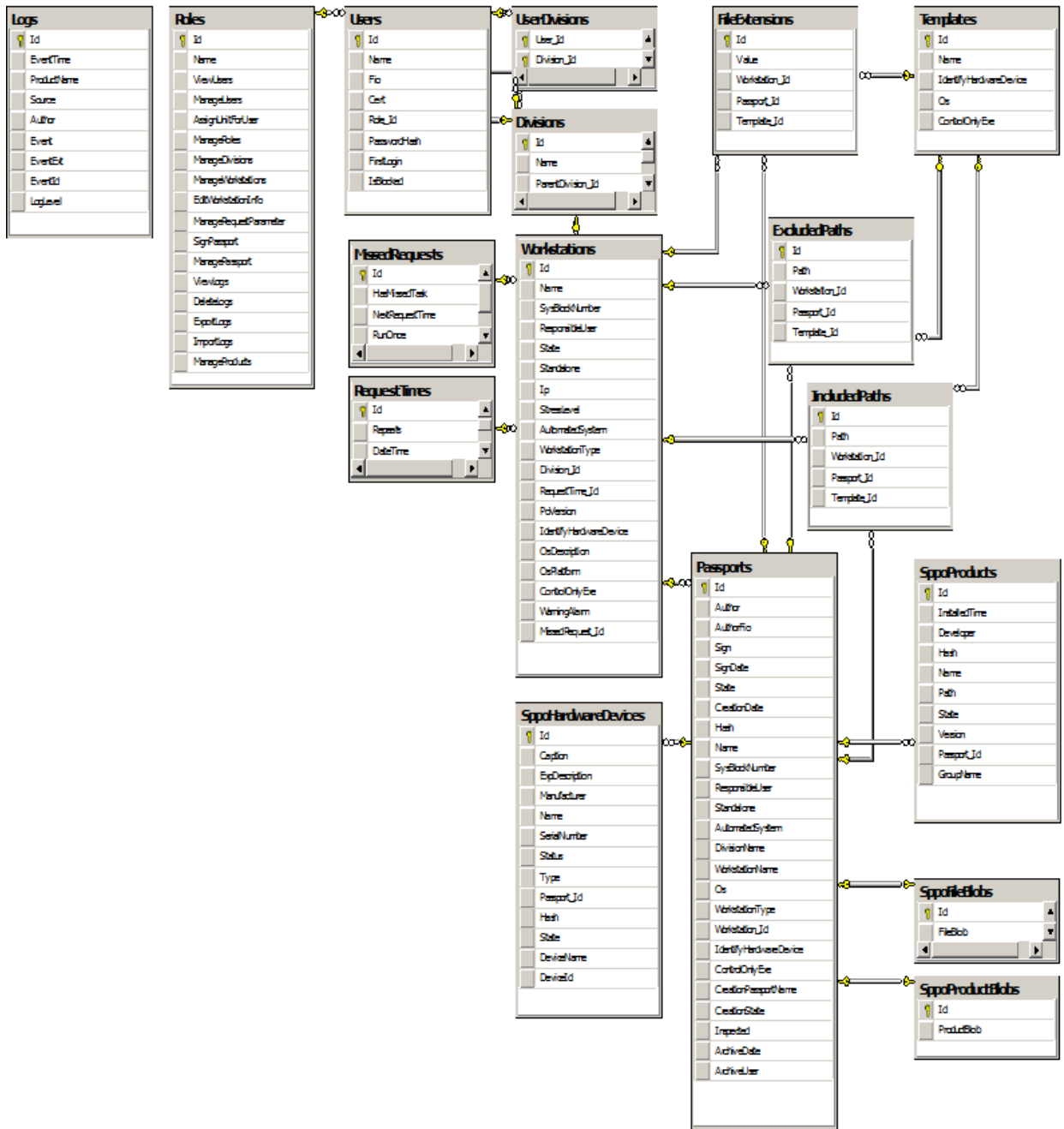
Рисунок 4 - Схема связей между таблицами базы данных ПМ «Паспорт ПО»
