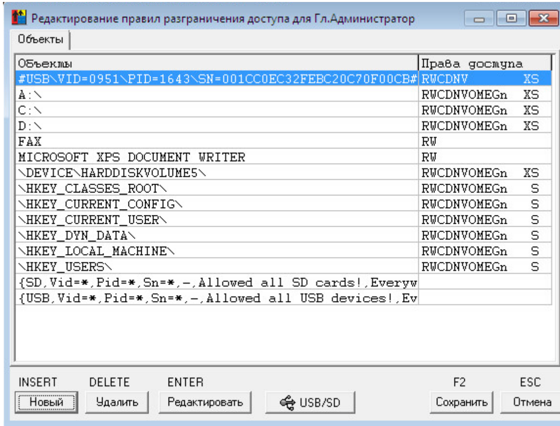
Рисунок 62 - Окно установки дискреционных ПРД к объектам
