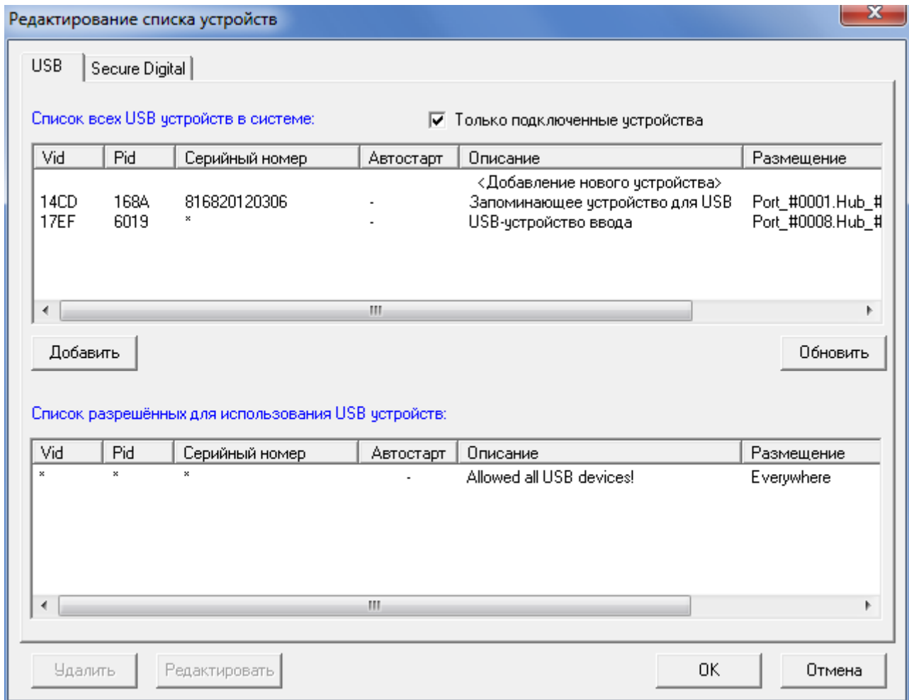
Рисунок 114 - Окно редактирования списка разрешенных устройств USB
