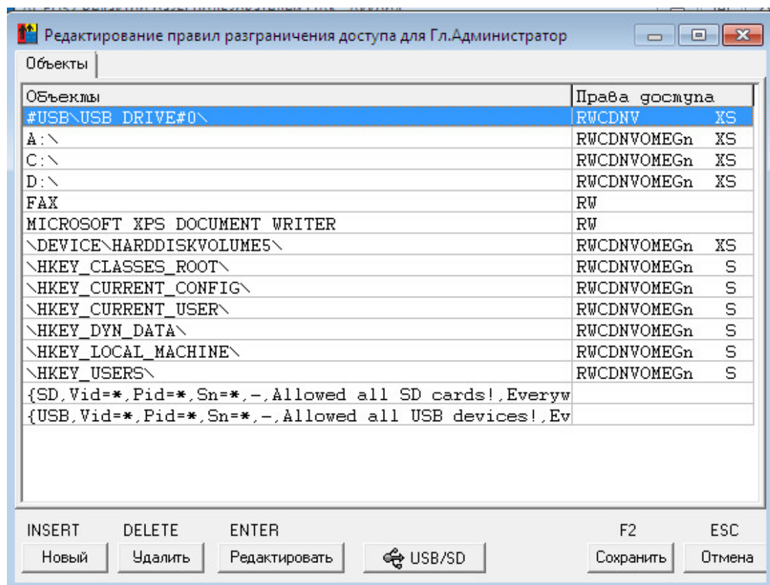
Рисунок 65 - Окно редактирования ПРД
