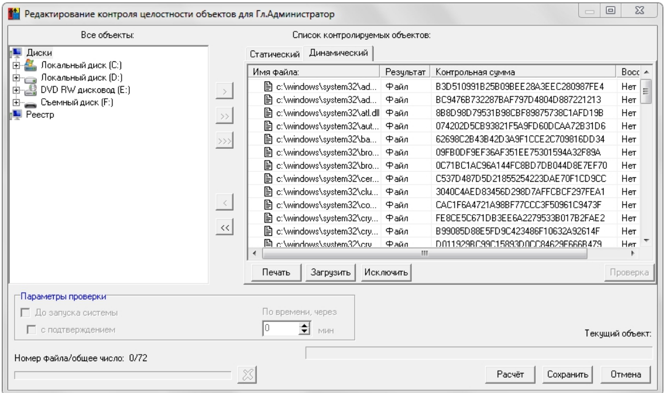
Рисунок 103 - Редактирование списков для контроля целостности. Контрольные суммы рассчитаны
