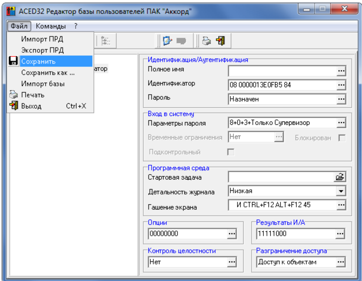
Рисунок 8 – Сохранение настроек
