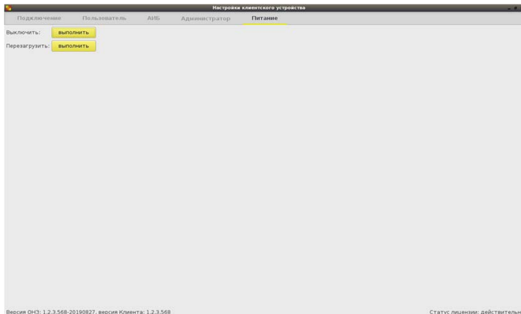
Рисунок 49 – Вкладка «Питание»
