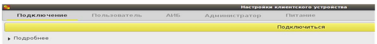
Рисунок 29 - Кнопка <Подключиться>
