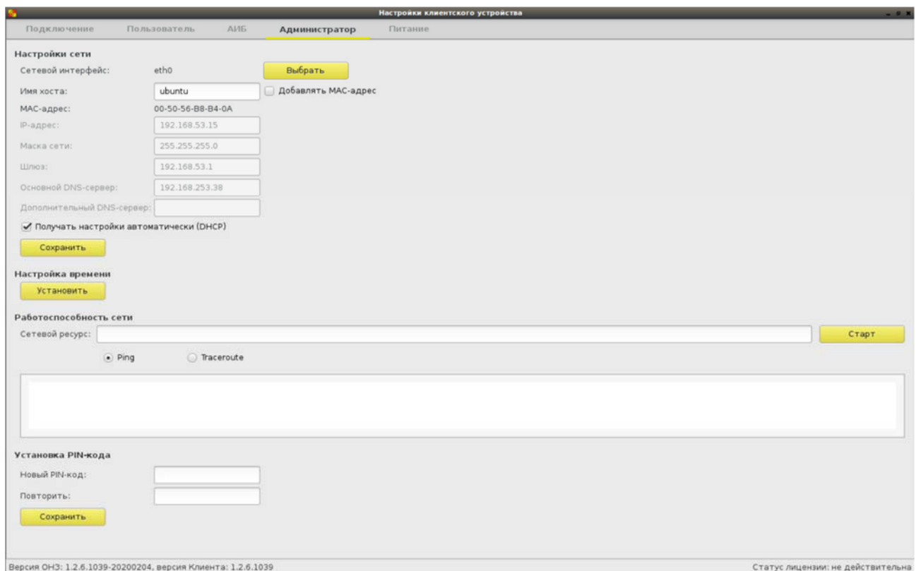
Рисунок 4 – Вкладка «Администратор»
