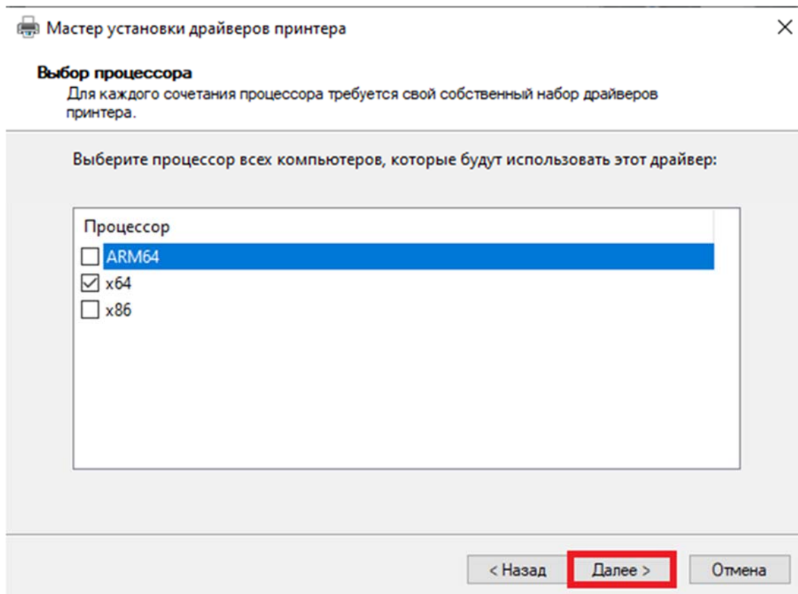
Рисунок 56 – Выбор процессора
