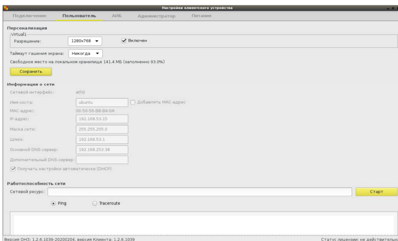
Рисунок 35 - Вкладка «Пользователь»
