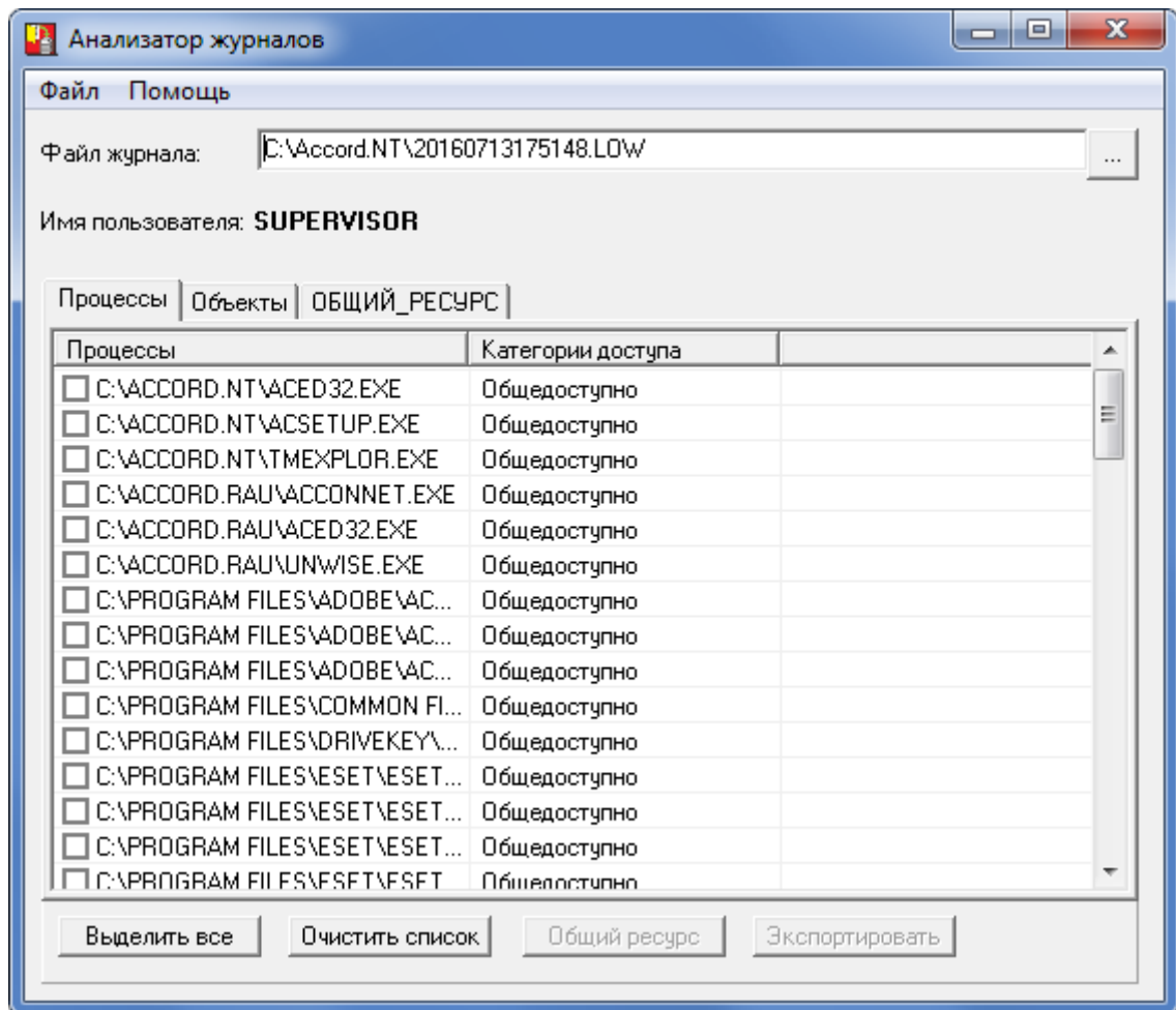
Рисунок 78 - Главное окно программы AcProc.exe. Выбор процесса
