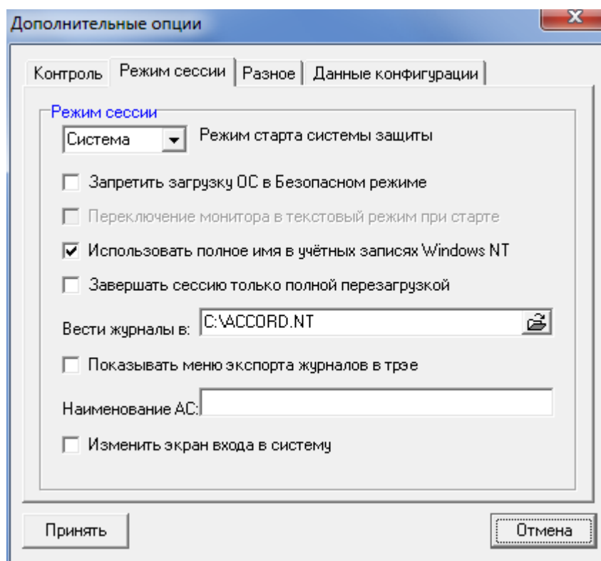
Рисунок 123 – Вкладка Настройка комплекса Аккорд\Дополнительные опции\Режим сессии
