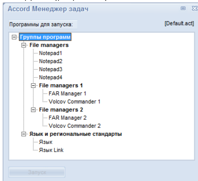
Рисунок 49 - Расположение задач в Менеджере задач при SortTask=1
