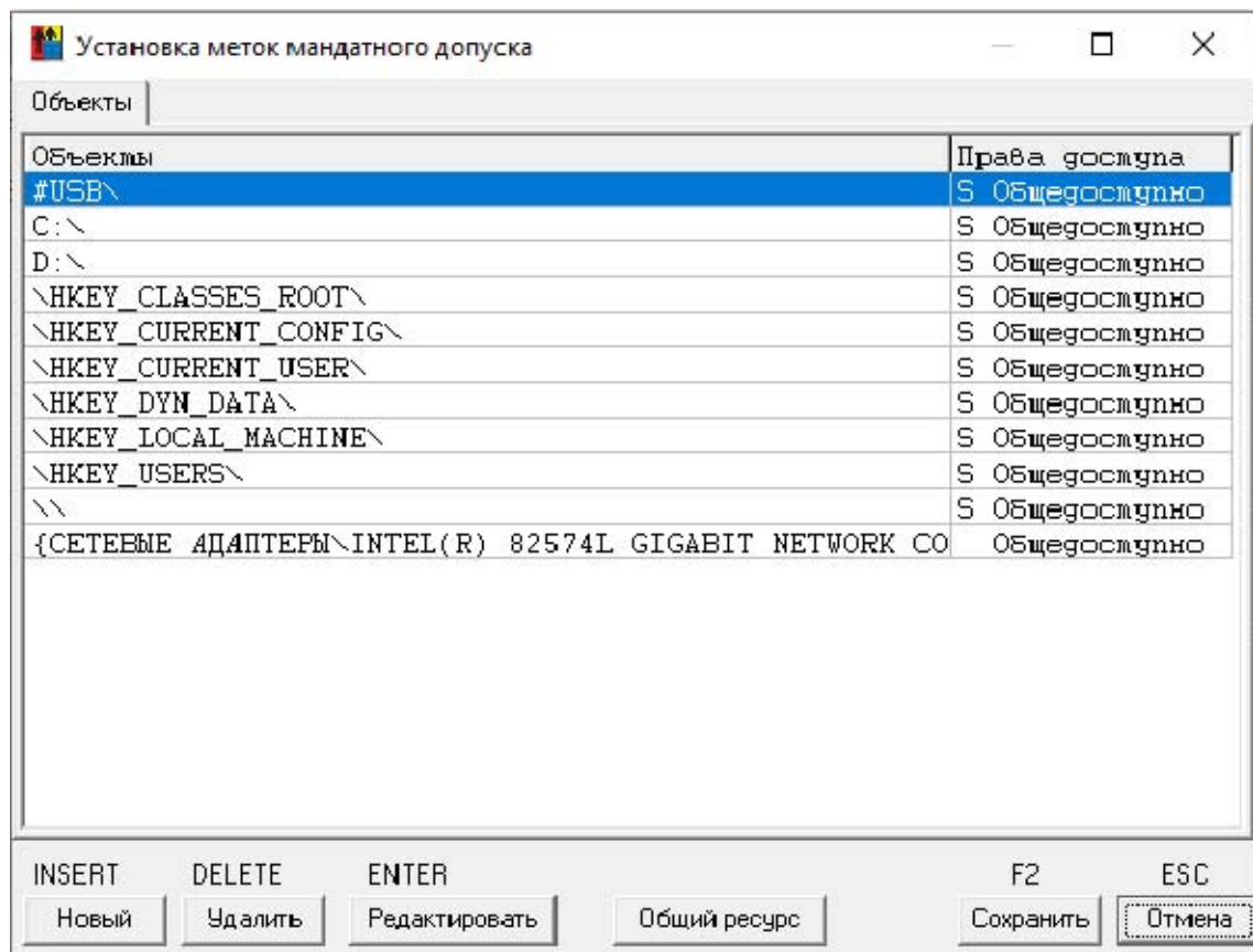
Рисунок 69 - Установка меток допуска объектов при использовании мандатных ПРД
