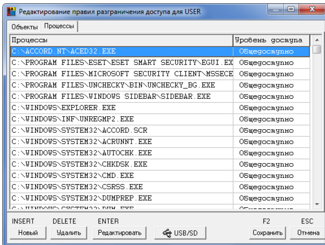
Рисунок 72 - Закладка «Процессы» при включенном механизме мандатного доступа для процессов
