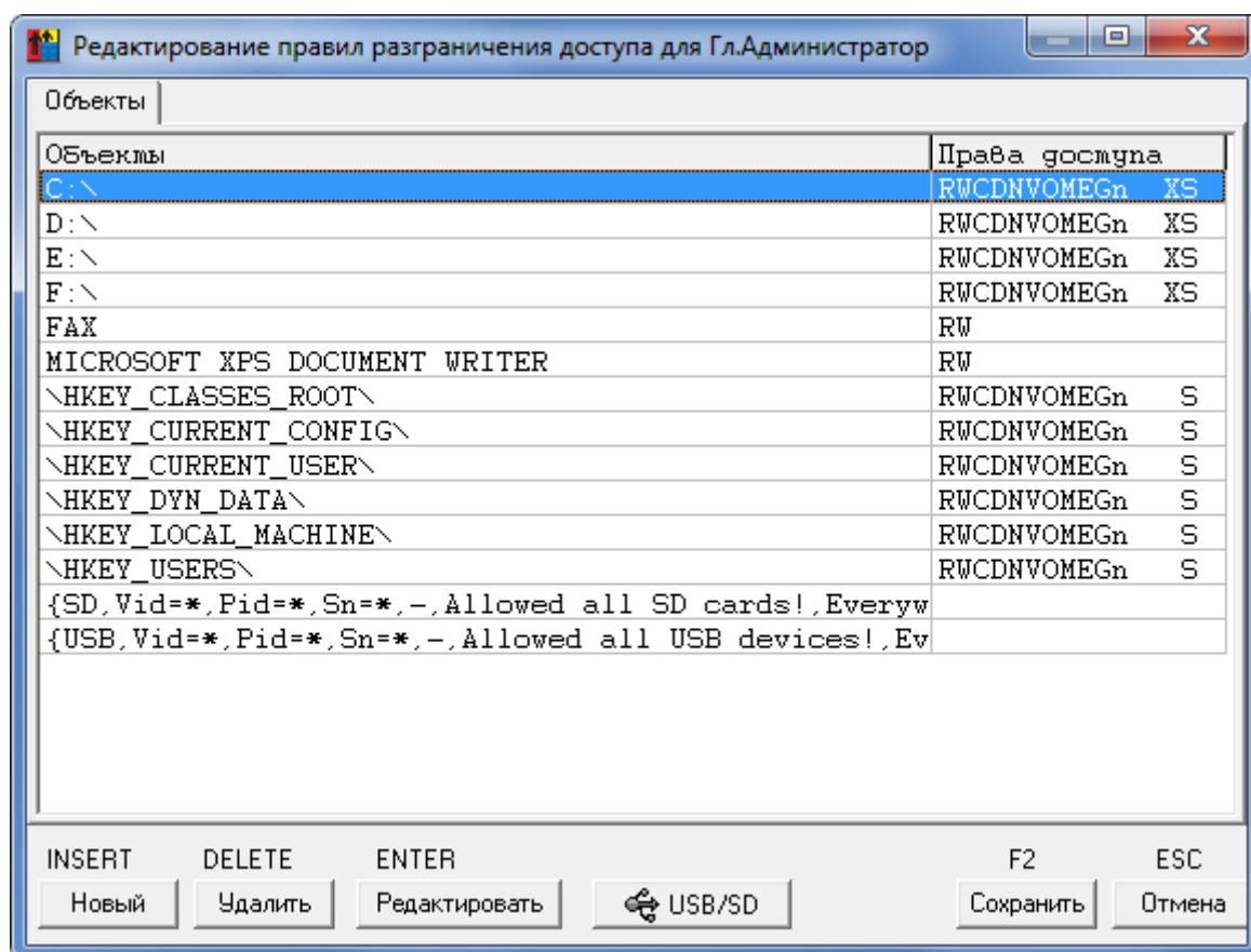
Рисунок 58 - Окно установки дискреционных ПРД к объектам
