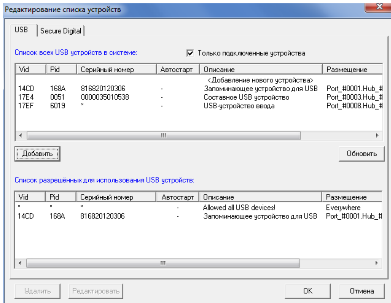
Рисунок 115 - USB устройство добавлено в список разрешенных
