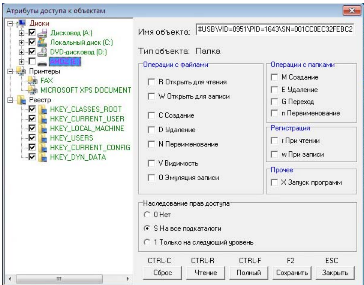
Рисунок 61 - Выбор USB-устройства и установка ПРД
