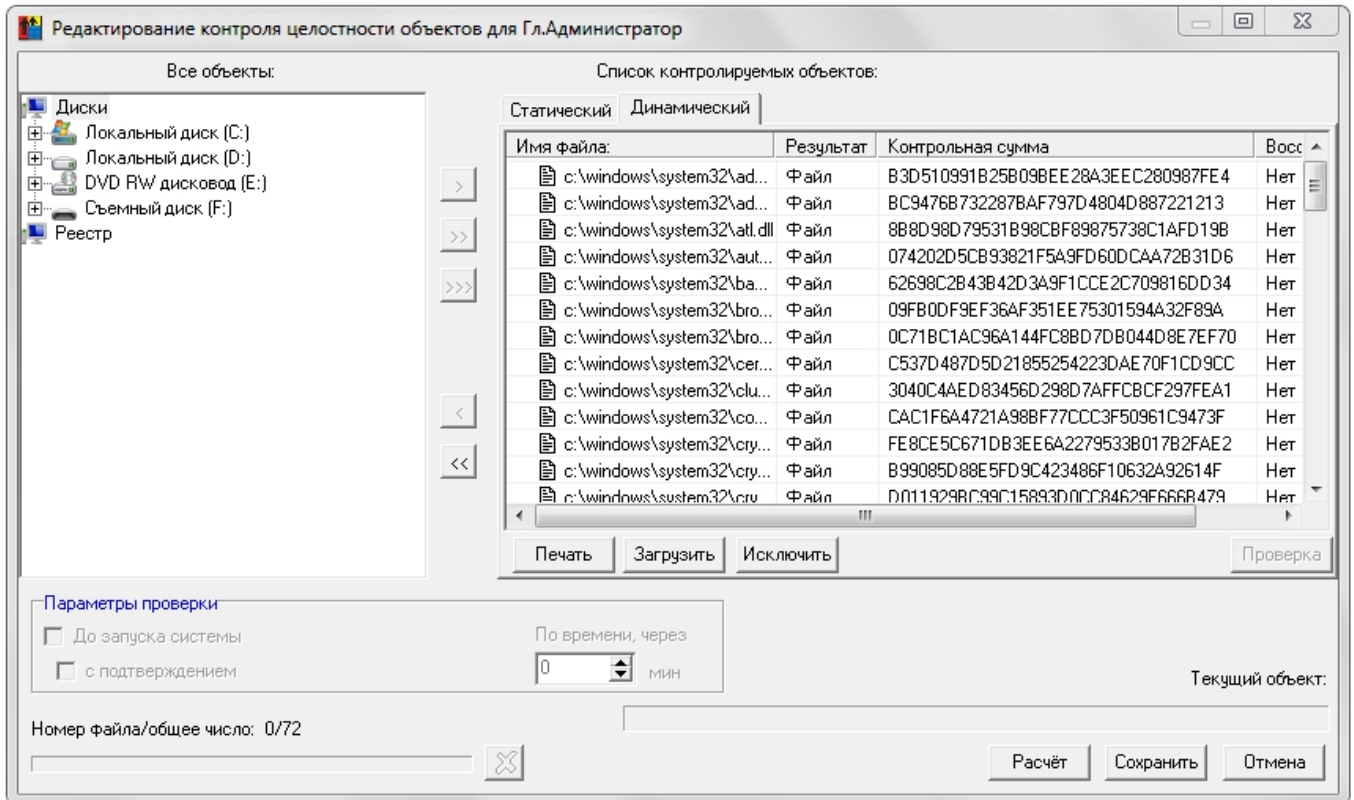
Рисунок 103 - Редактирование списков для контроля целостности. Контрольные суммы рассчитаны
