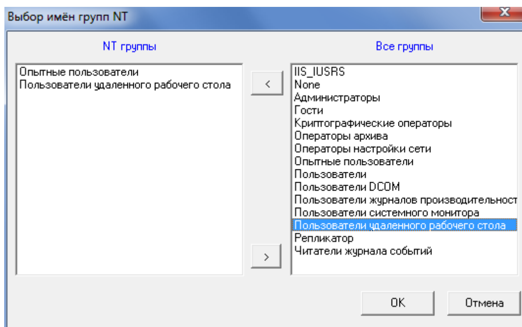
Рисунок 121 - Синхронизация пользователя СЗИ «Аккорд» с несколькими группами ОС
