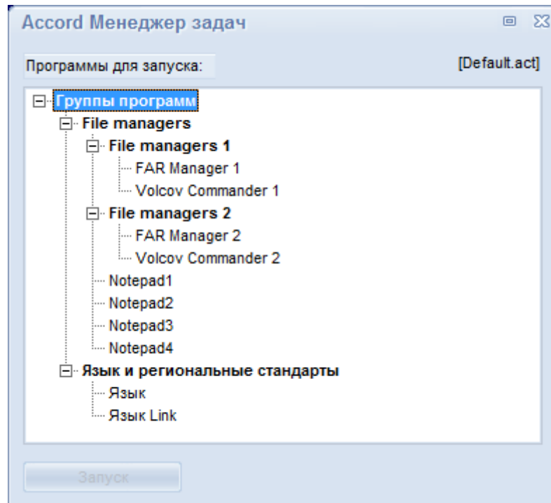
Рисунок 48 - Расположение задач в Менеджере задач при SortTask=0
