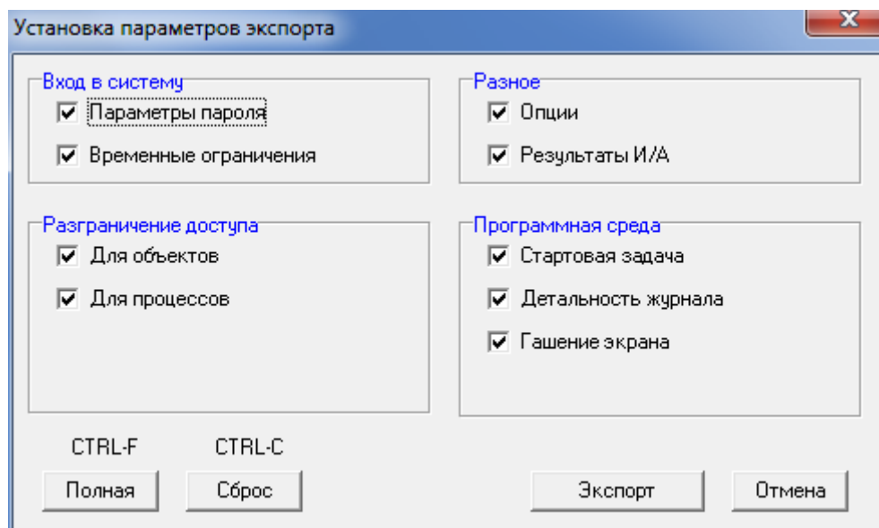
Рисунок 109 - Выбор параметров ПРД для экспорта
