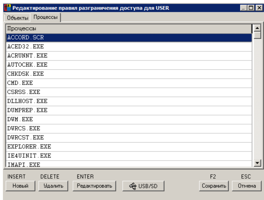
Рисунок 99 - Список импортированных процессов (дискреционный механизм разграничения доступа)
