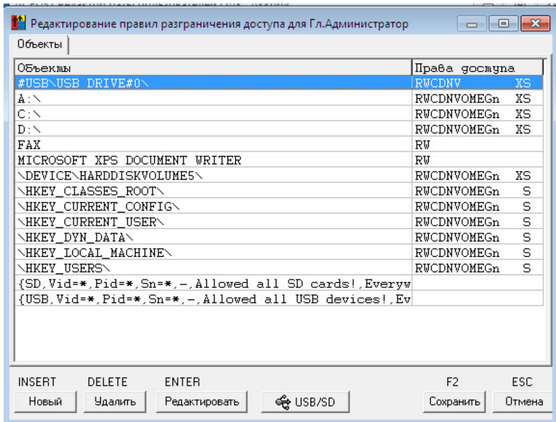
Рисунок 65 - Окно редактирования ПРД
