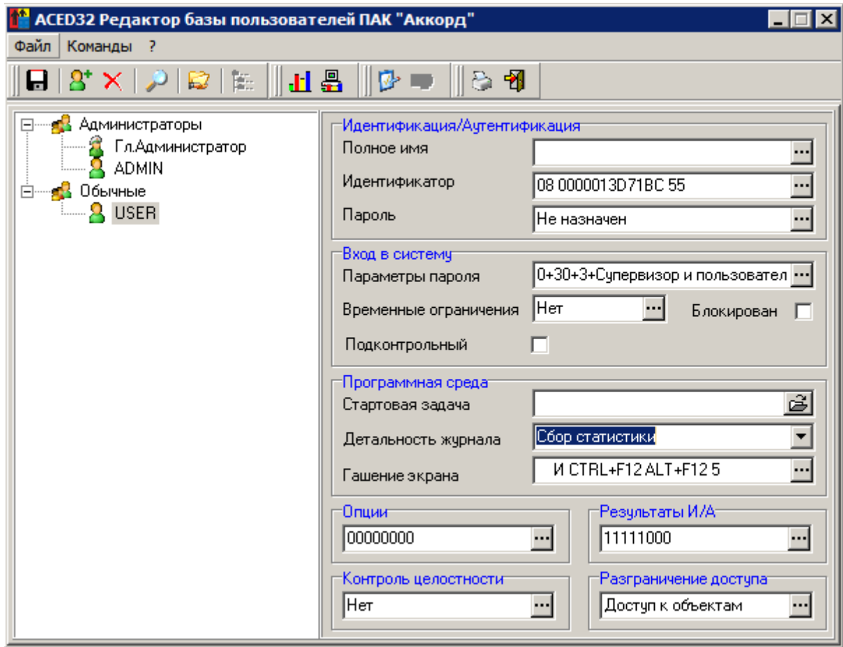
Рисунок 83 - Установка уровня детальности журнала «Сбор статистики»
