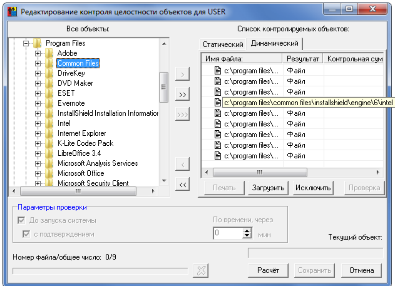
Рисунок 54 - Список файлов для динамического контроля
