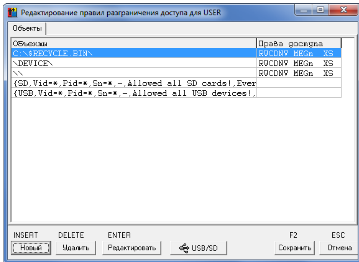
Рисунок 129 – Список доступа Startup-пользователя
