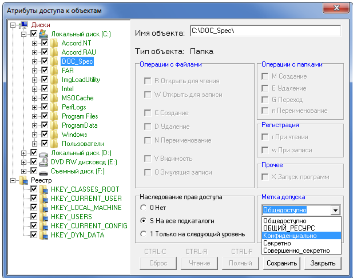
Рисунок 70 - Определение нового объекта и выбор его метки допуска
