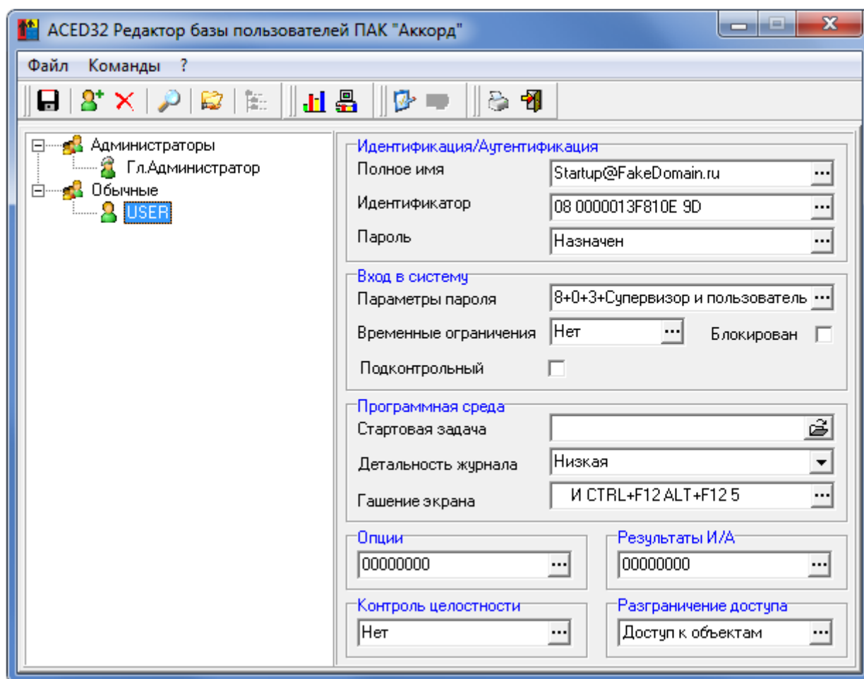
Рисунок 124 – Главное окно редактора прав доступа. Задание полного имени Startup-пользователя
