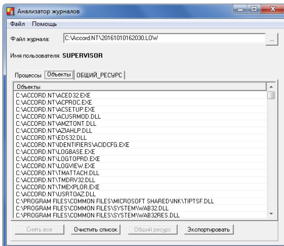
Рисунок 92 – Главное окно программы АсПроc.exe. Вкладка «Объекты»
