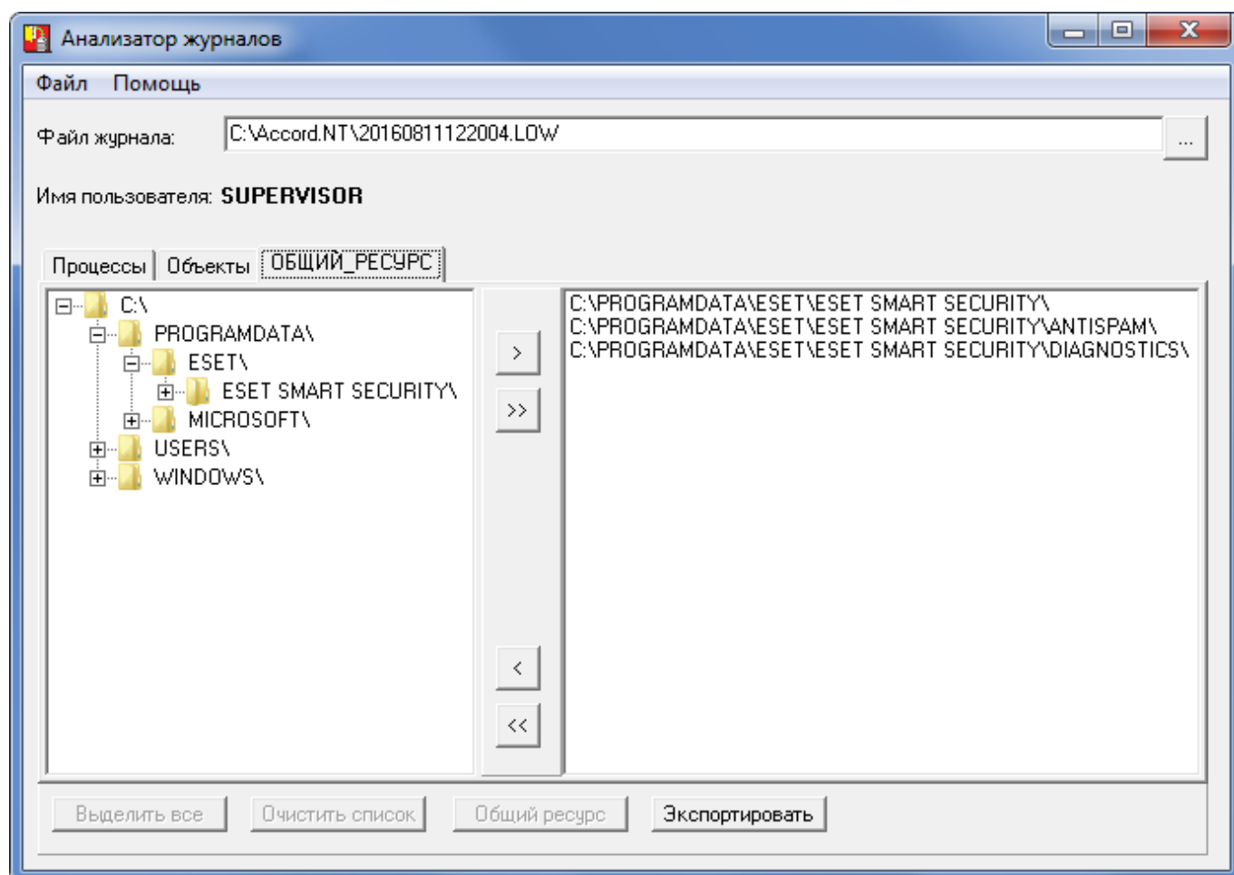
Рисунок 79 – Список объектов общего доступа
