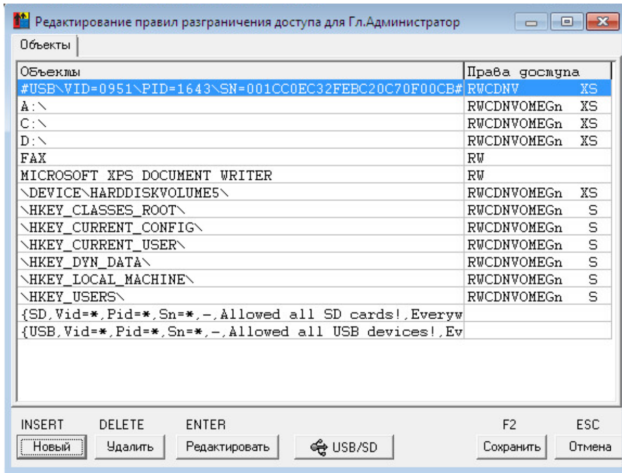
Рисунок 62 - Окно установки дискреционных ПРД к объектам
