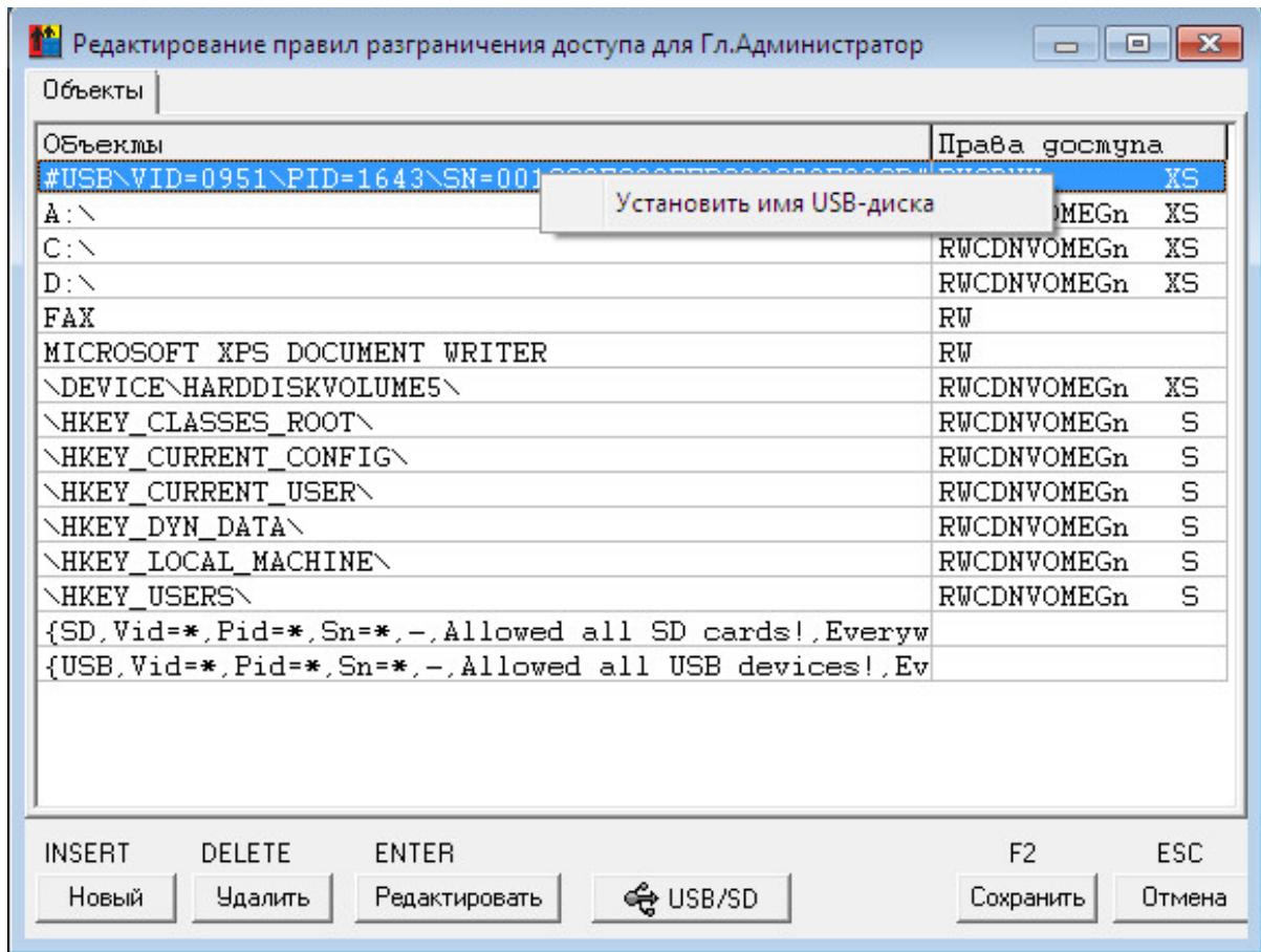
Рисунок 63 - Окно редактирования ПРД
