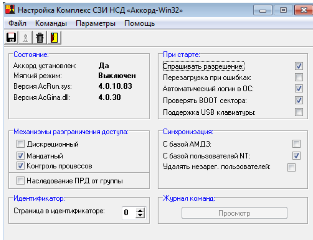
Рисунок 57 - – Главное окно утилиты «Настройка комплекса Аккорд»
