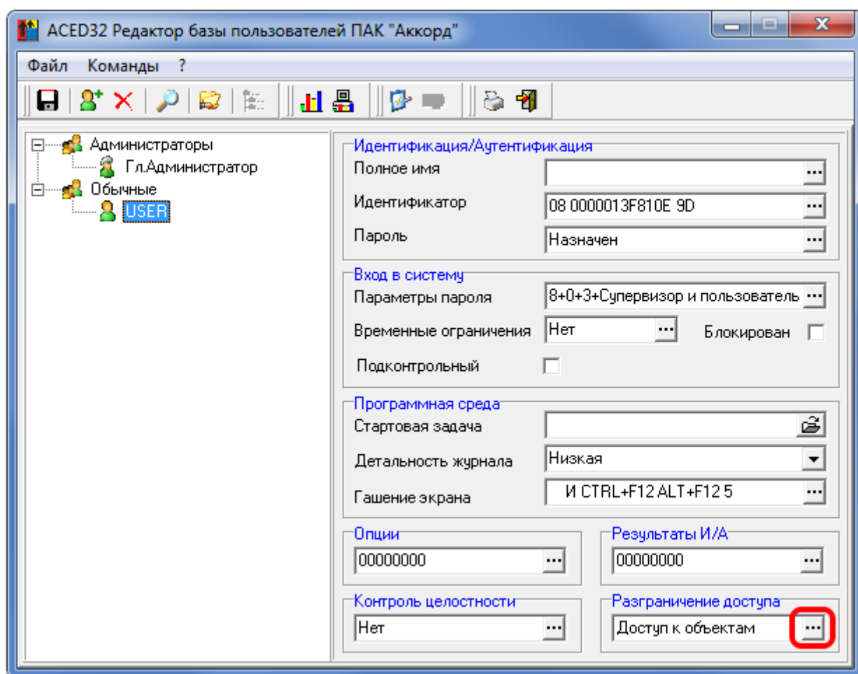
Рисунок 125 – Главное окно редактора прав доступа. Выбор меню разграничения доступа для Startup-пользователя
