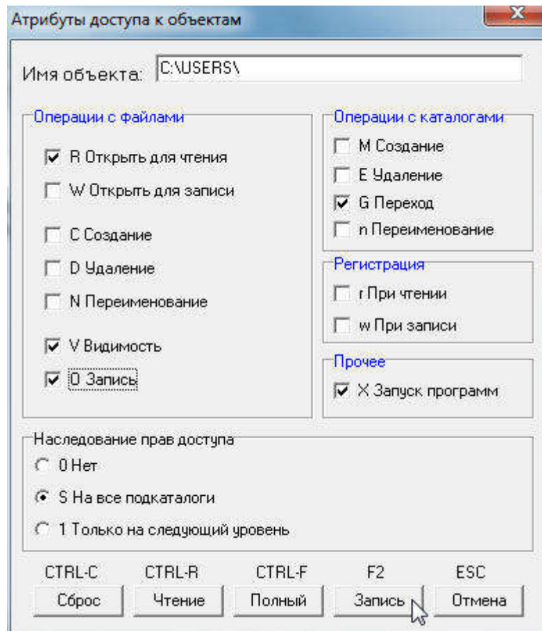
Рисунок 24 - Окно установки атрибутов доступа
