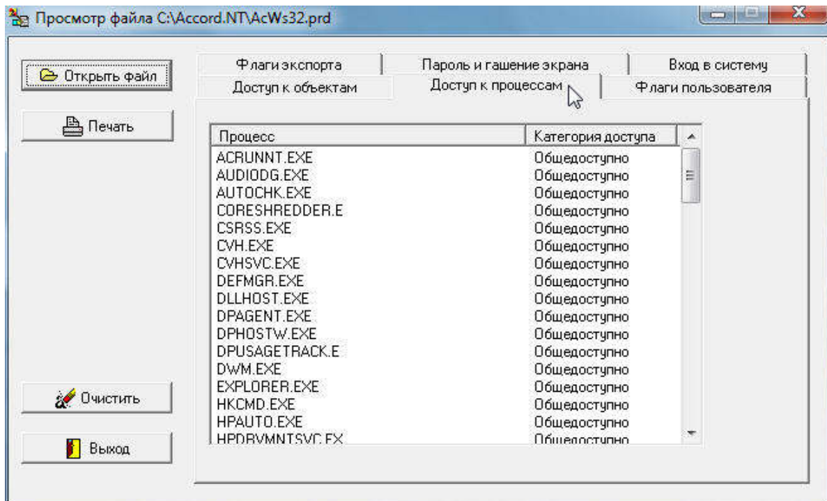
Рисунок 37 - Данные о правилах доступа и настройках пользователя
