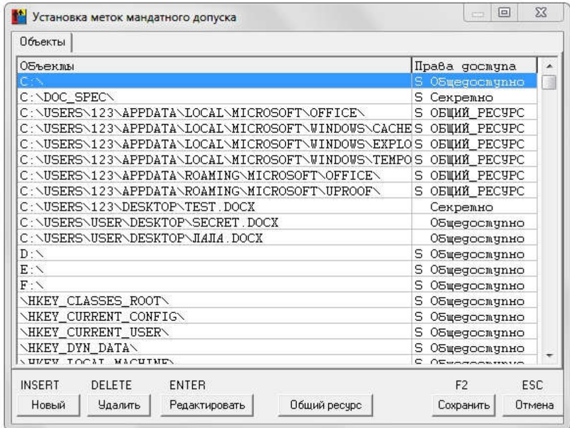
Рисунок 35 - Список объектов с метками мандатного доступа
