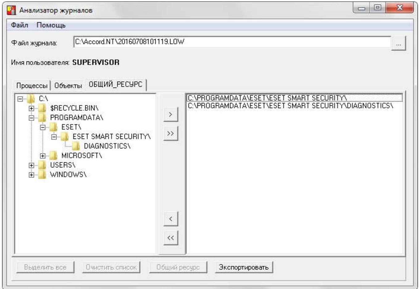
Рисунок 32 - Выбор процесса для исследования
