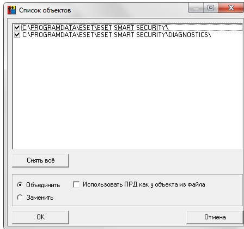
Рисунок 34 - Список объектов в процедуре импорта
