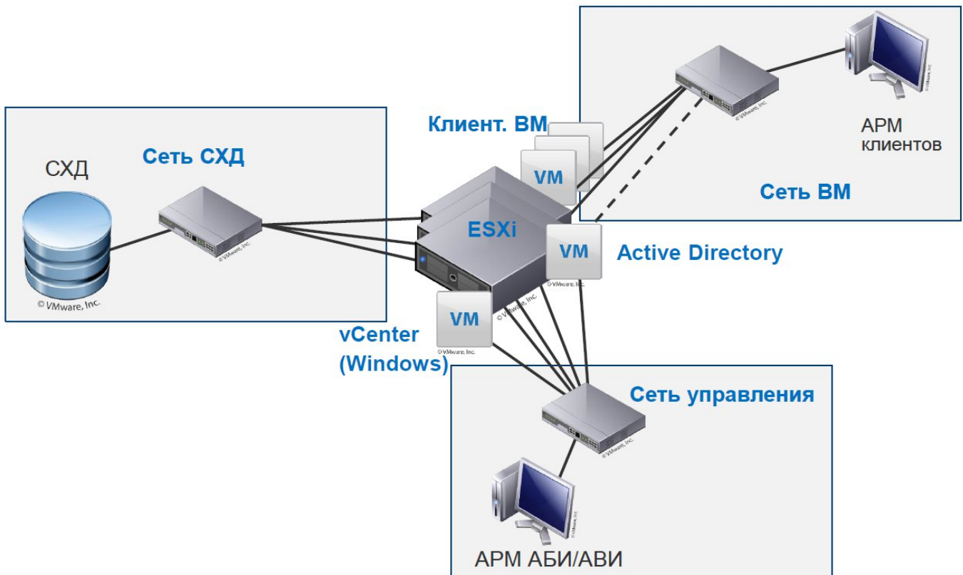
Рисунок 1 - Пример разворачиваемой инфраструктуры
