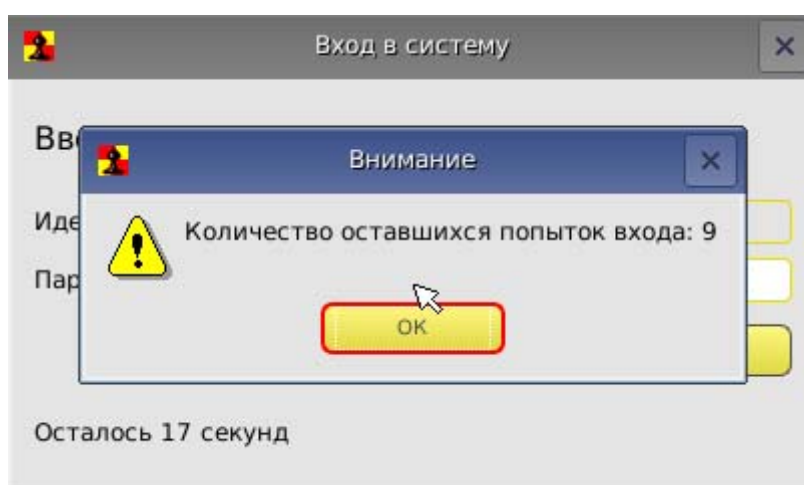
Рисунок 7 – Предупреждающее сообщение
