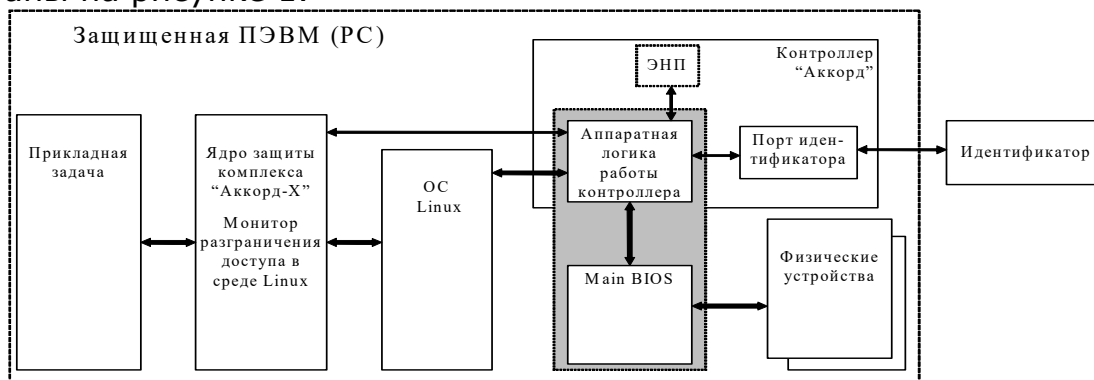
Рисунок 1. Схема построения системы защиты информации
