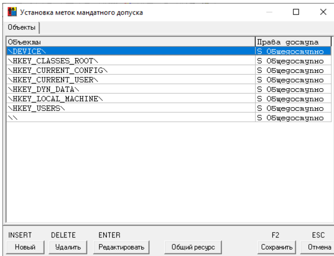
Рисунок 33 – Установка меток мандатного допуска
