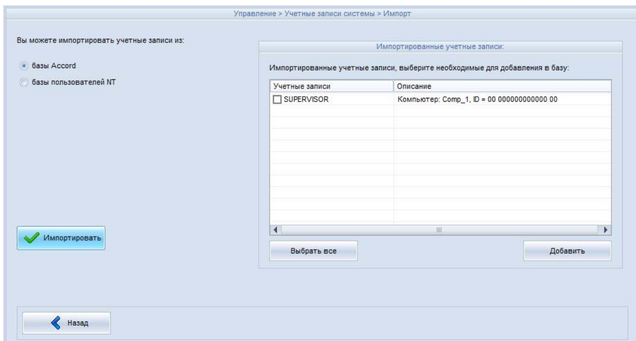
Рисунок 82 - Выбор импортированных учетных записей (импорт из базы «Аккорда»)
