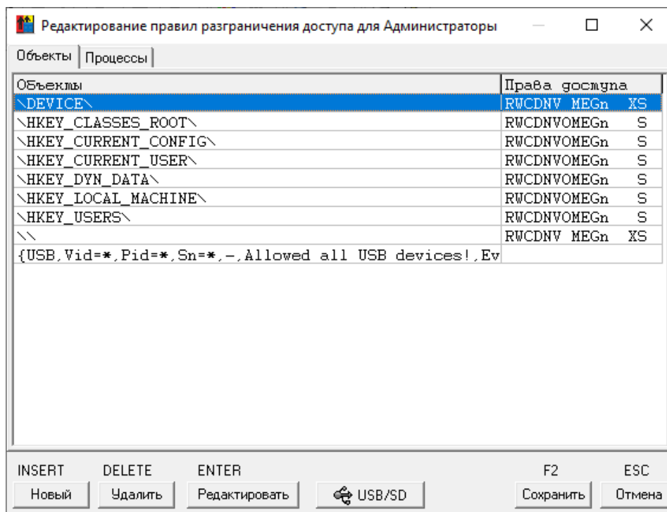
Рисунок 14 – Перечень объектов для установки прав доступа
