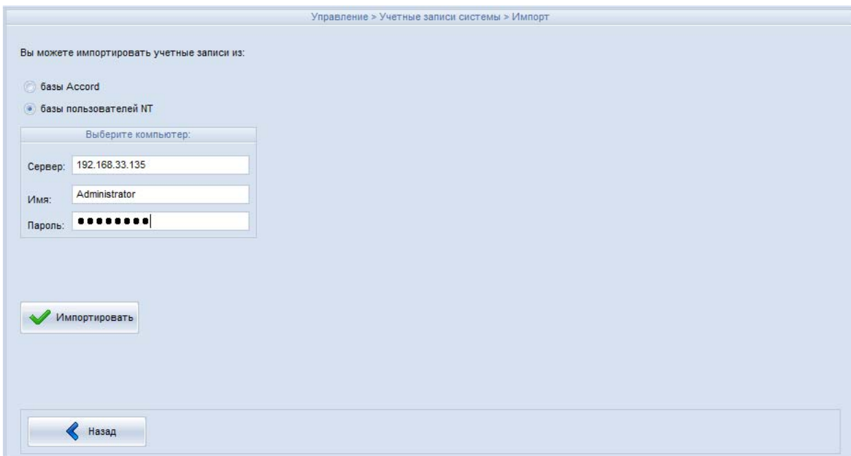
Рисунок 77 - Ввод данных о сервере, из базы пользователей которого будут импортированы учетные записи
