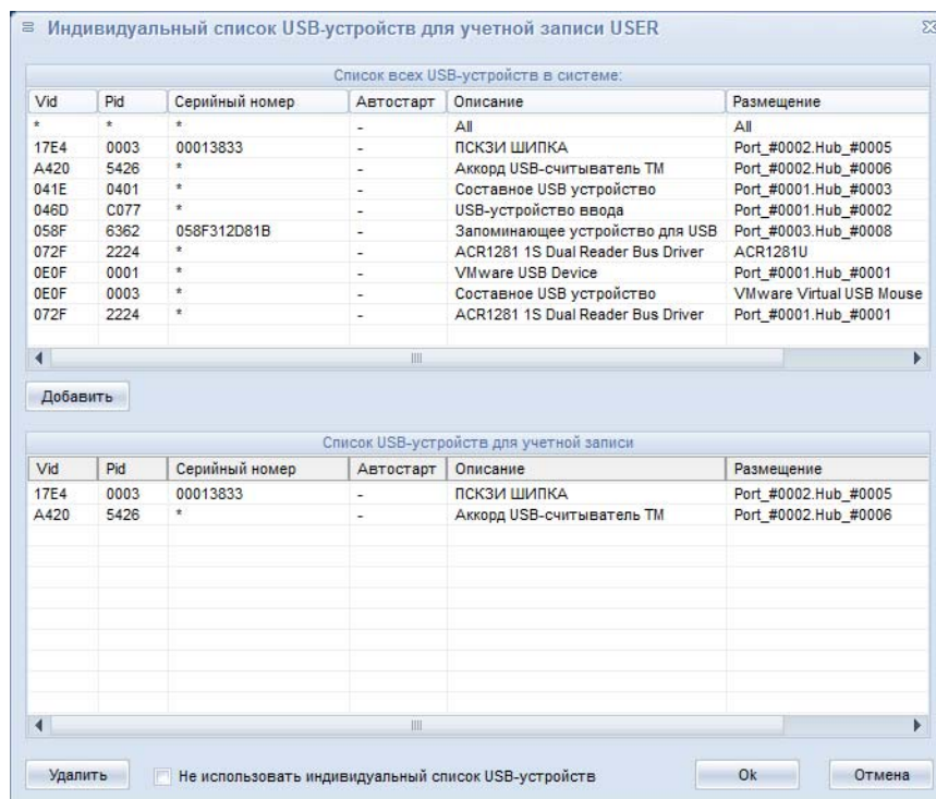
Рисунок 66 - Настройка списка разрешённых USB-устройств для учётной записи
