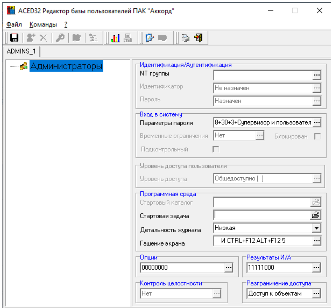
Рисунок 13 – Редактирование базы пользователей «Аккорд»
