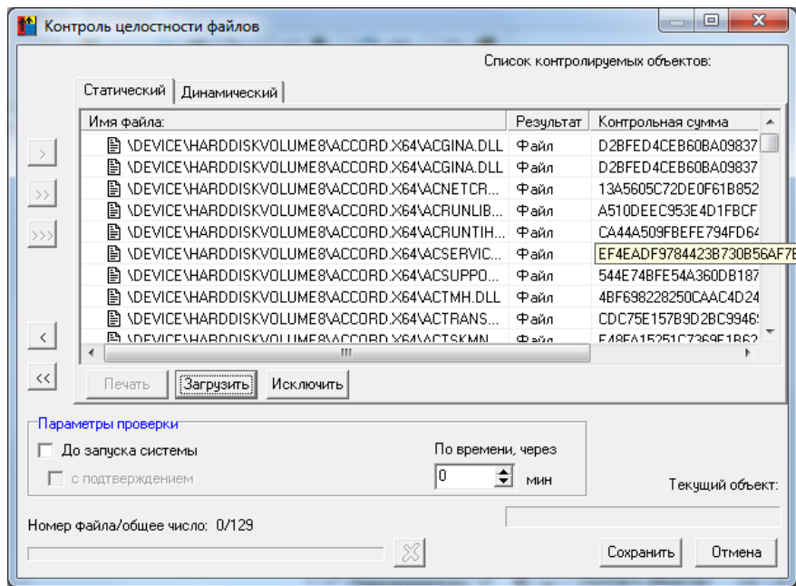
Рисунок 60 - Список файлов, целостность которых контролируется на ПКО
