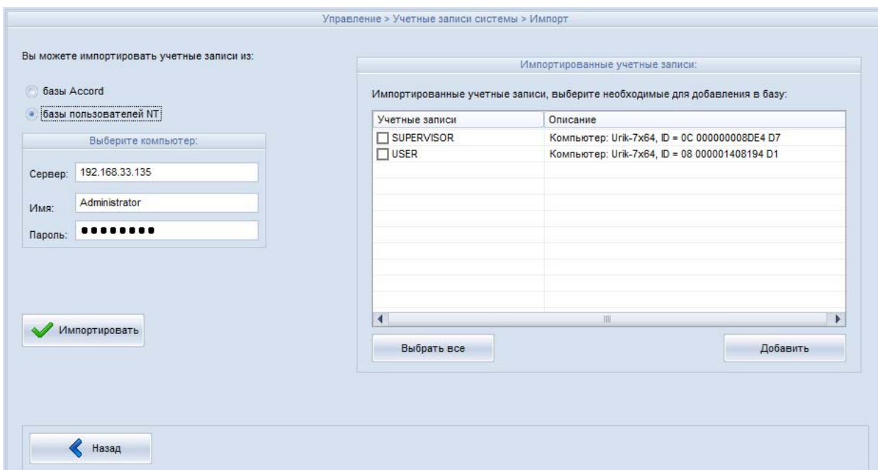
Рисунок 78 - Выбор импортированных учетных записей (импорт из базы пользователей NT)
