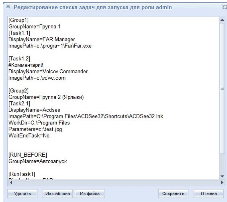
Рисунок 8 – Редактирование списка задач для запуска
