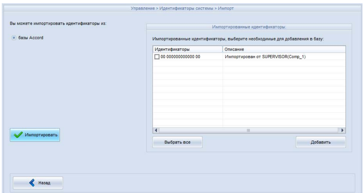
Рисунок 24 - Выбор импортированных идентификаторов (импорт из базы «Аккорда»)
