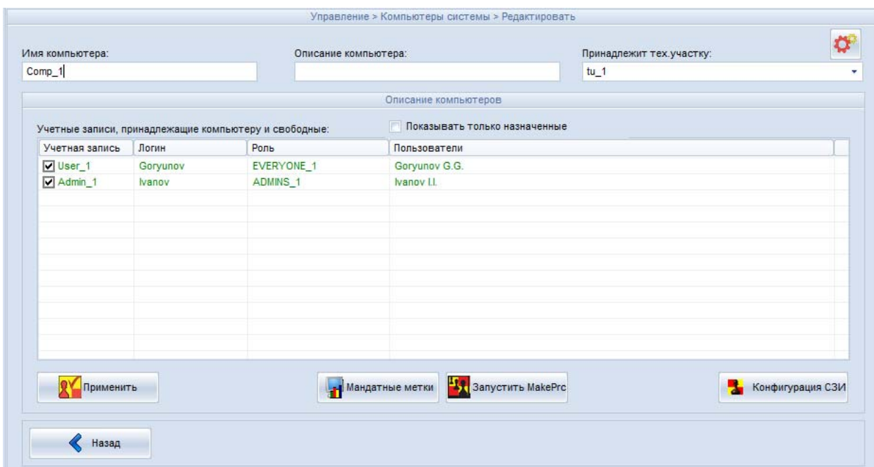
Рисунок 32 – Редактирование списка подконтрольных объектов
