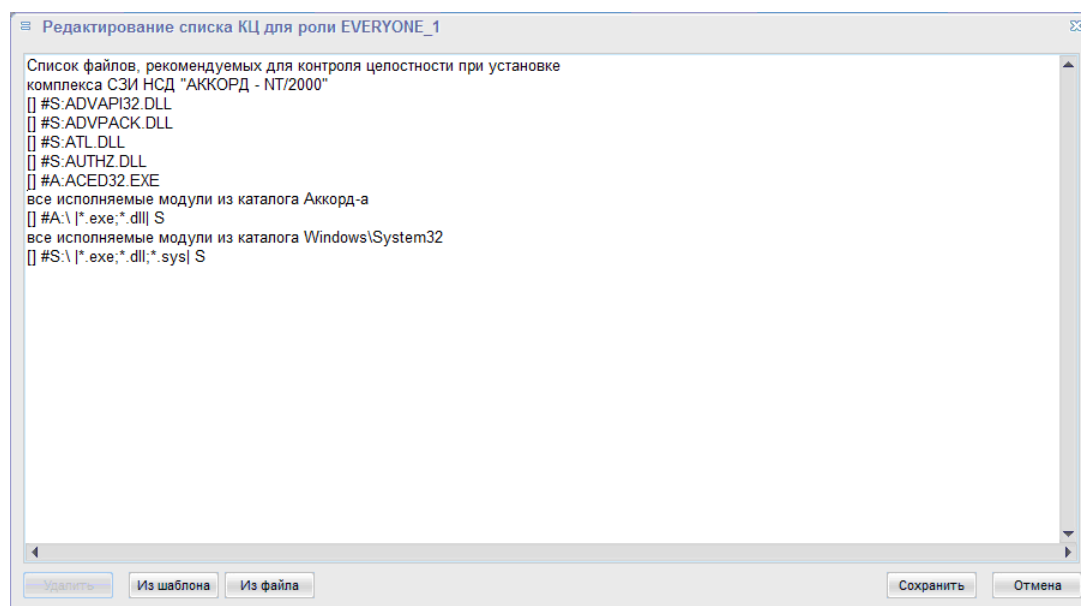
Рисунок 10 - Редактирование списка контролируемых файлов
