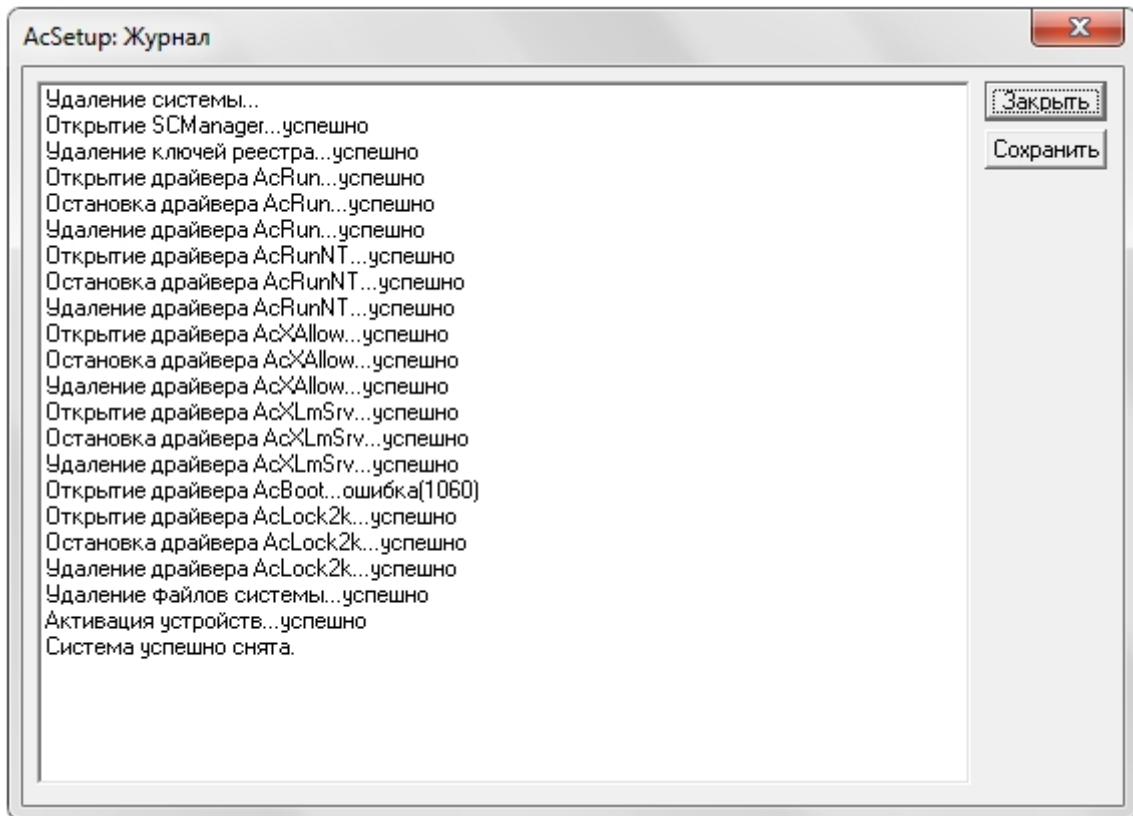
Рисунок 13 – Просмотр журнала команд утилиты AcSetup.EXE
