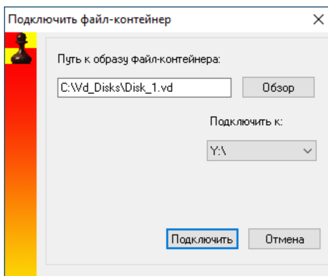
Рисунок 29 - Подключение файла-контейнера
