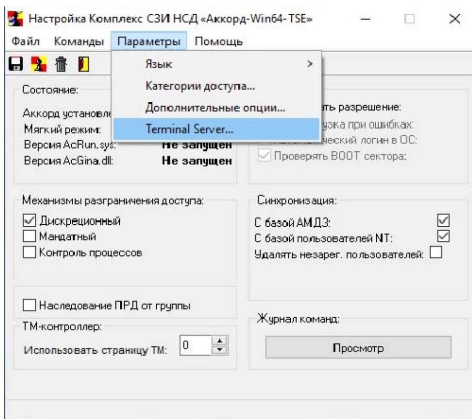
Рисунок 34 - Пункт меню «Terminal Server» в программе настройки комплекса
