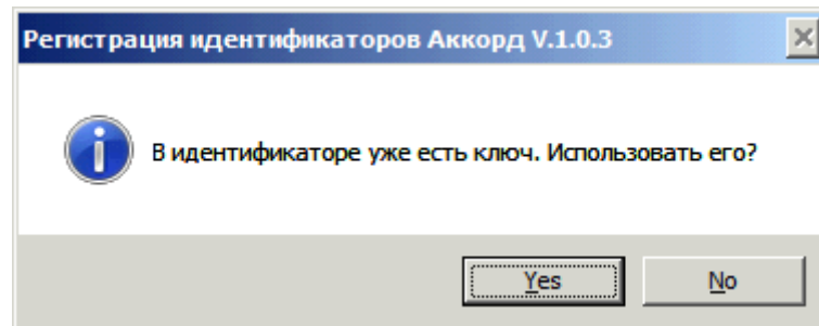
Рисунок 44 – Регистрация идентификатора
