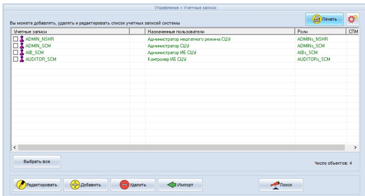
Рисунок 4 - Вкладка Управление > Учётные записи
