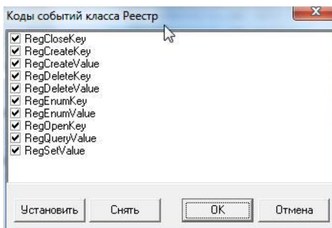
Рисунок 10 - Установка фильтра для событий класса «Реестр»
